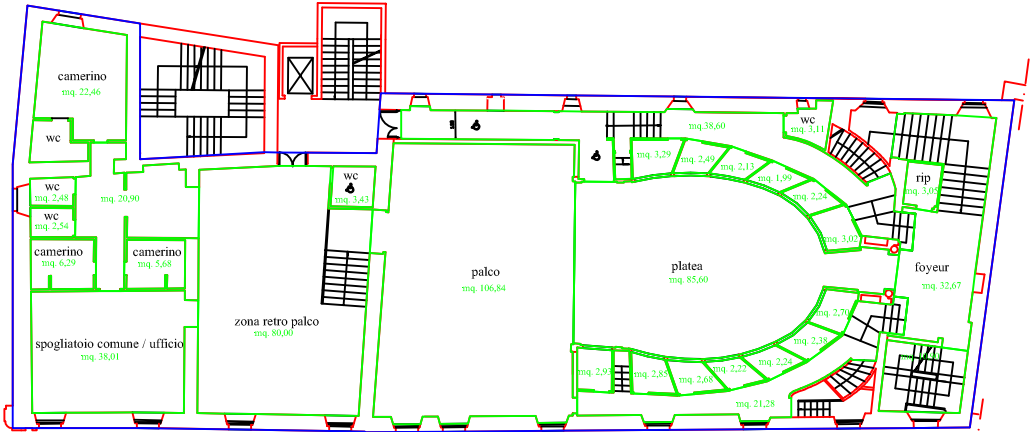
PIANO PLATEA - 1° ORDINE - CAMERINI Sup. Utile mq. 516,40 Sup. Lorda mq. 645,33
