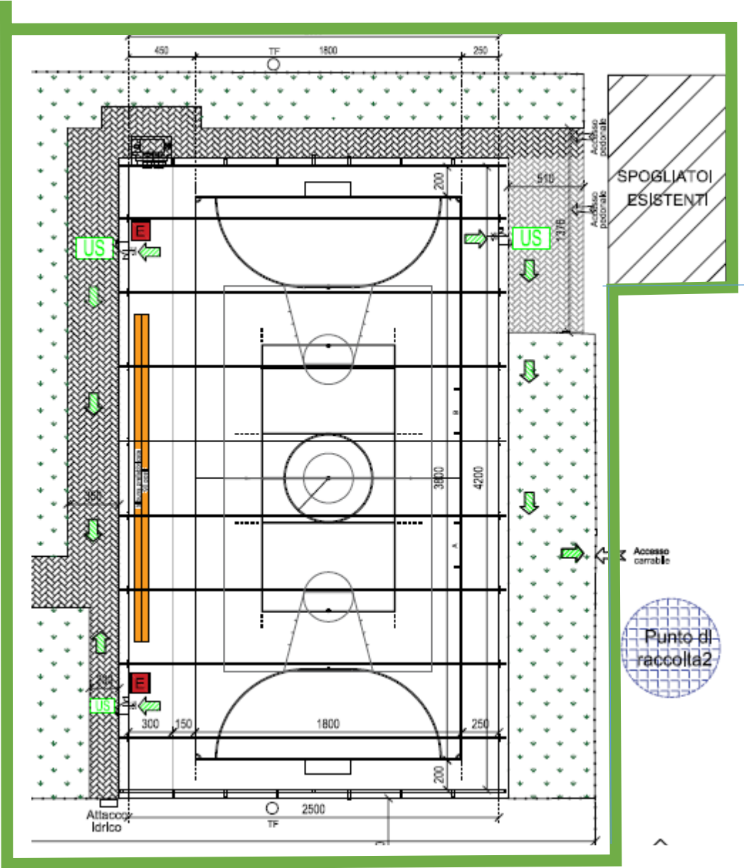
Allegato 1 - Planimetria Generale
