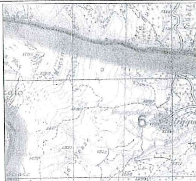
Carta dei terreni sottoposti a vincolo per scopi idrogeologici R.D. n. 3267/1923 Estratto Carta IGM - Scala 1:25.000
