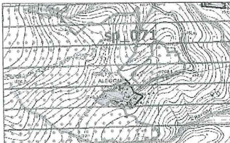
Piano Territoriale Paesistico Regionale Beni del patrimonio naturale e culturale artt. 21, 22 e 23 L.R. 24/98 Estratto Tavola COS foglio 337
