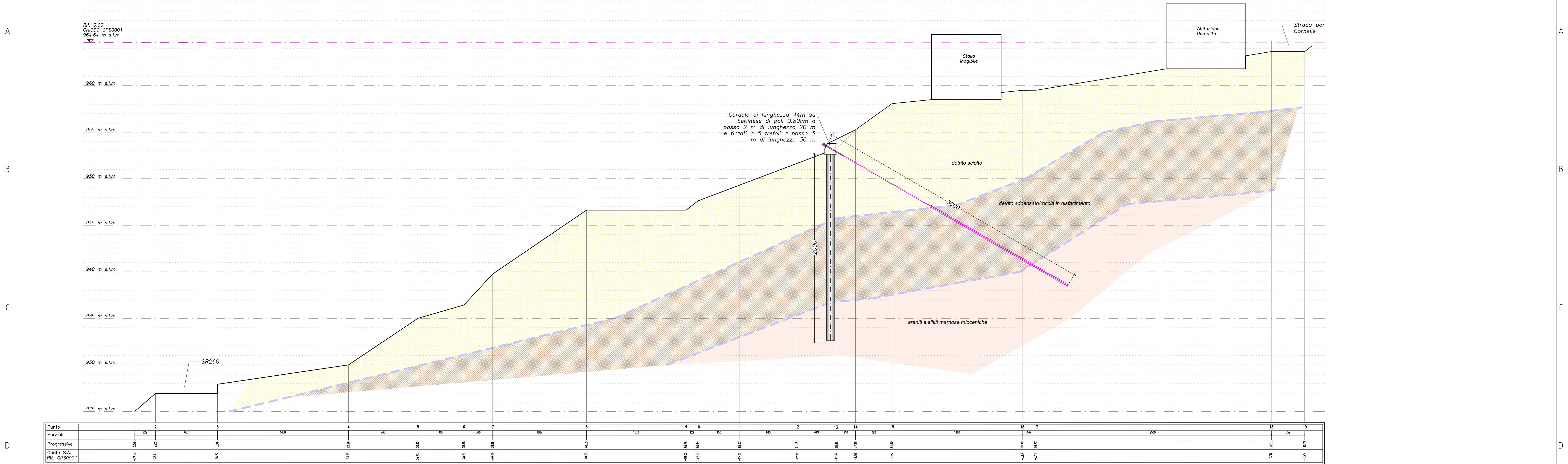
Sezione 2 - scala 1:200
