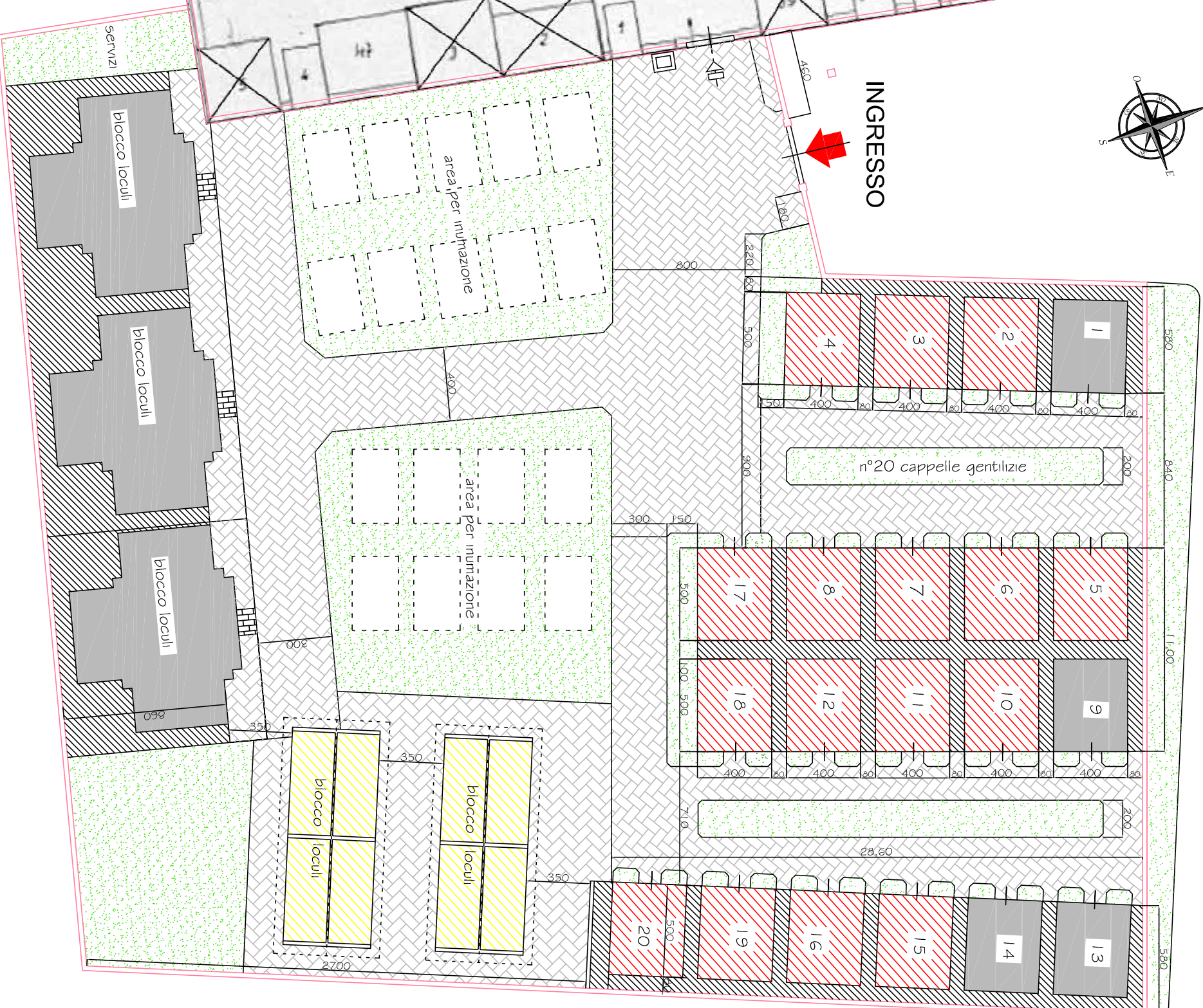
Cimitero frazione San Lorenzo a Flaviano - Planimetria generale
