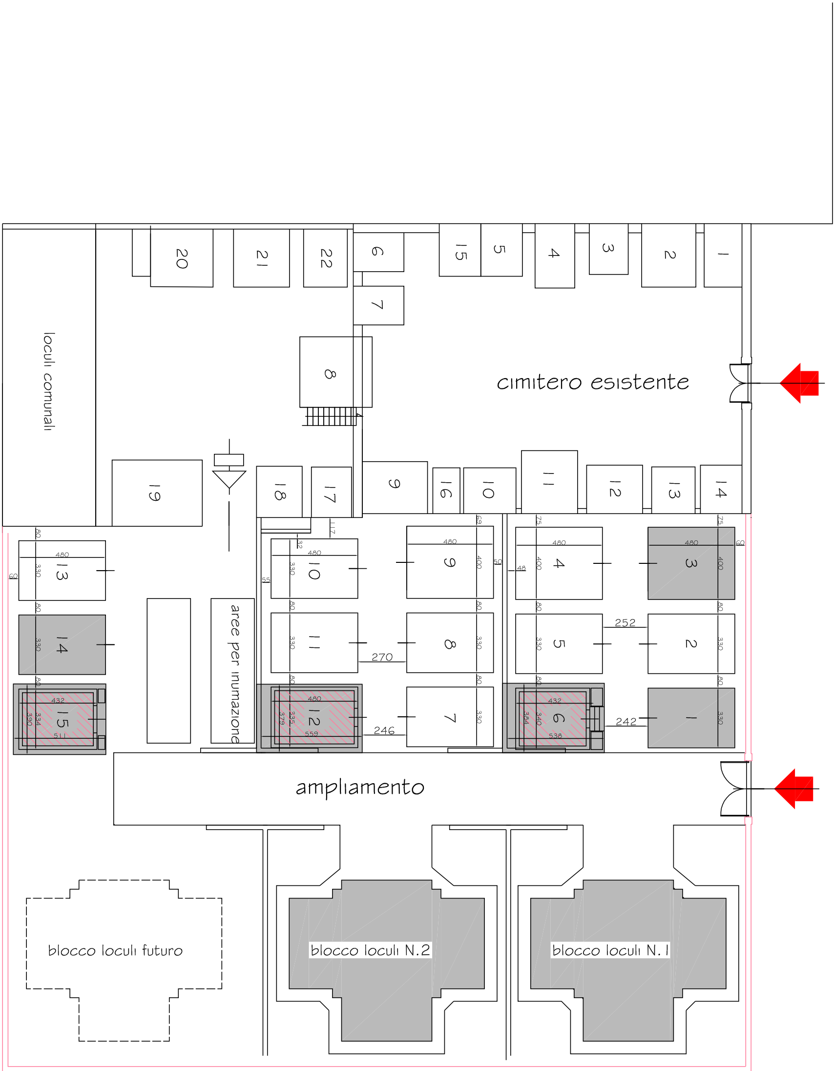
Cimitero frazione Nommisci - Planimetria generale ampliamento
