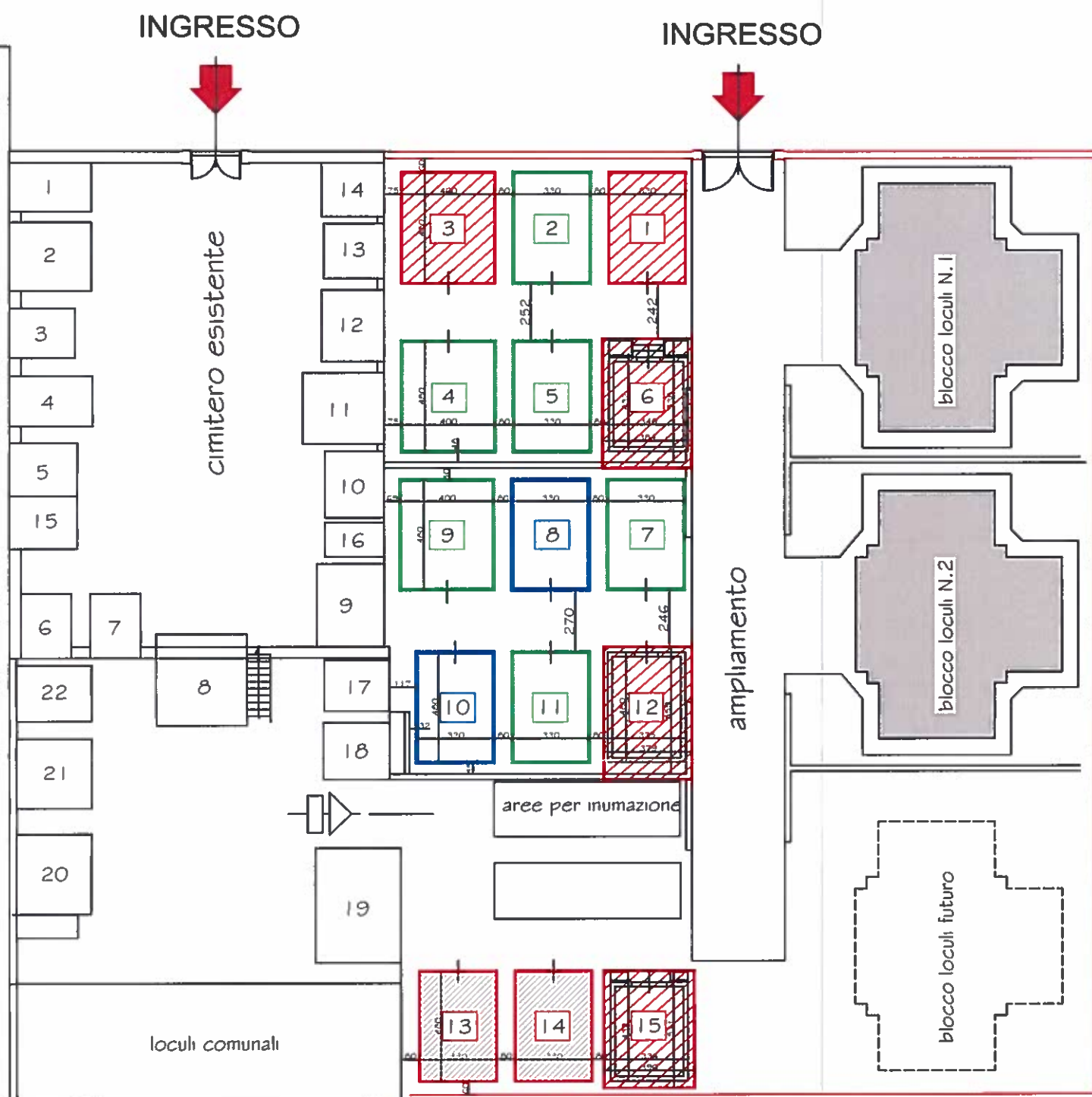
Cimitero frazione Nommisci - Planimetria generale ampliamento
