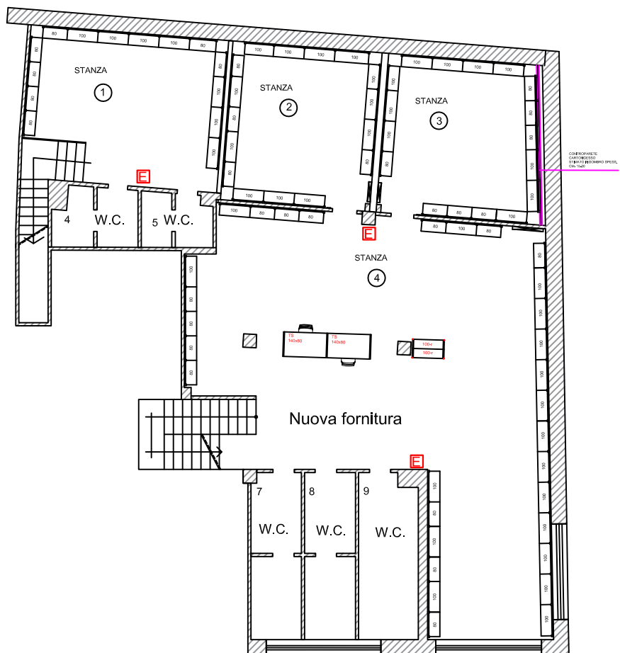
PIANTA PIANO INTERRATO
