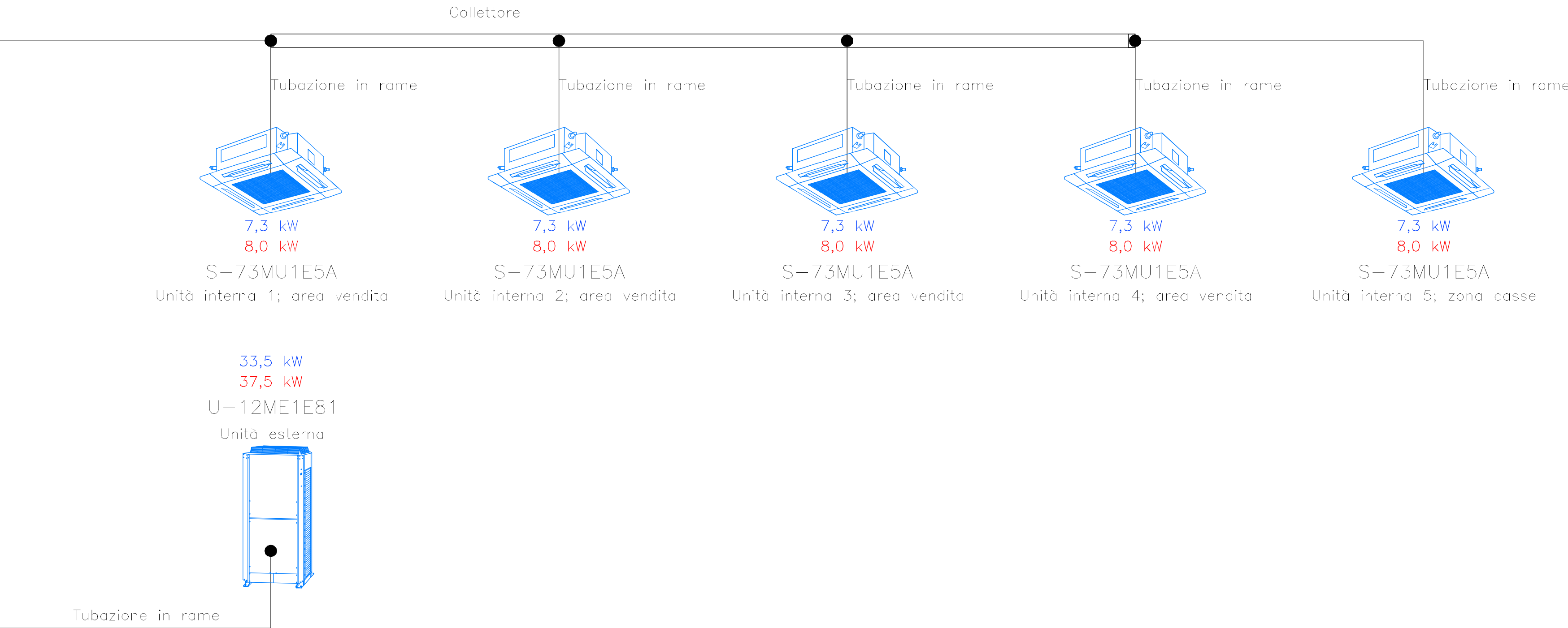
SCHEMA FUNZIONALE IMPIANTO DI CLIMATIZZAZIONE
