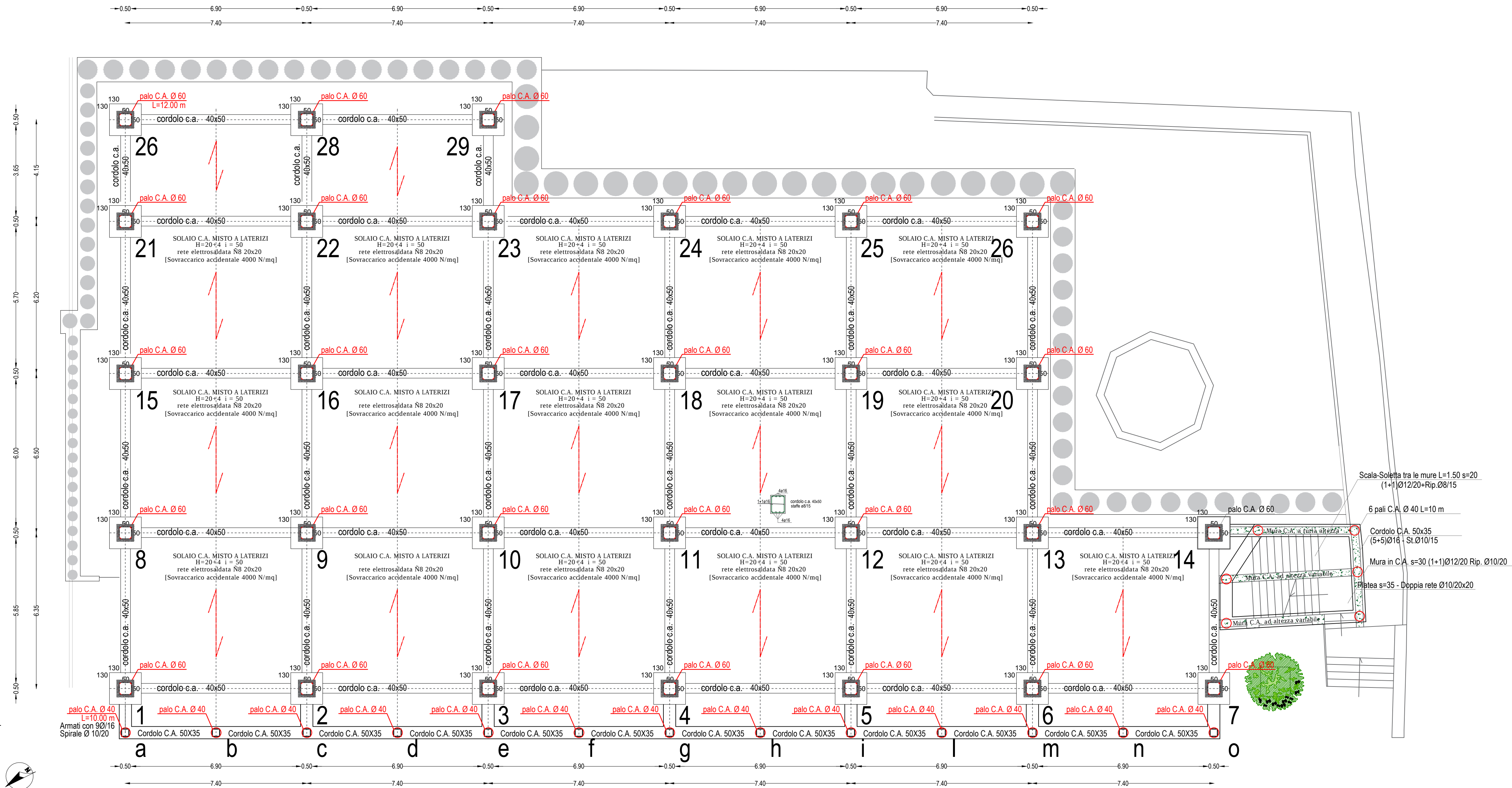
PIANTA FONDAZIONI e 1° SOLAIO FONDAZIONE - SC 1.100
