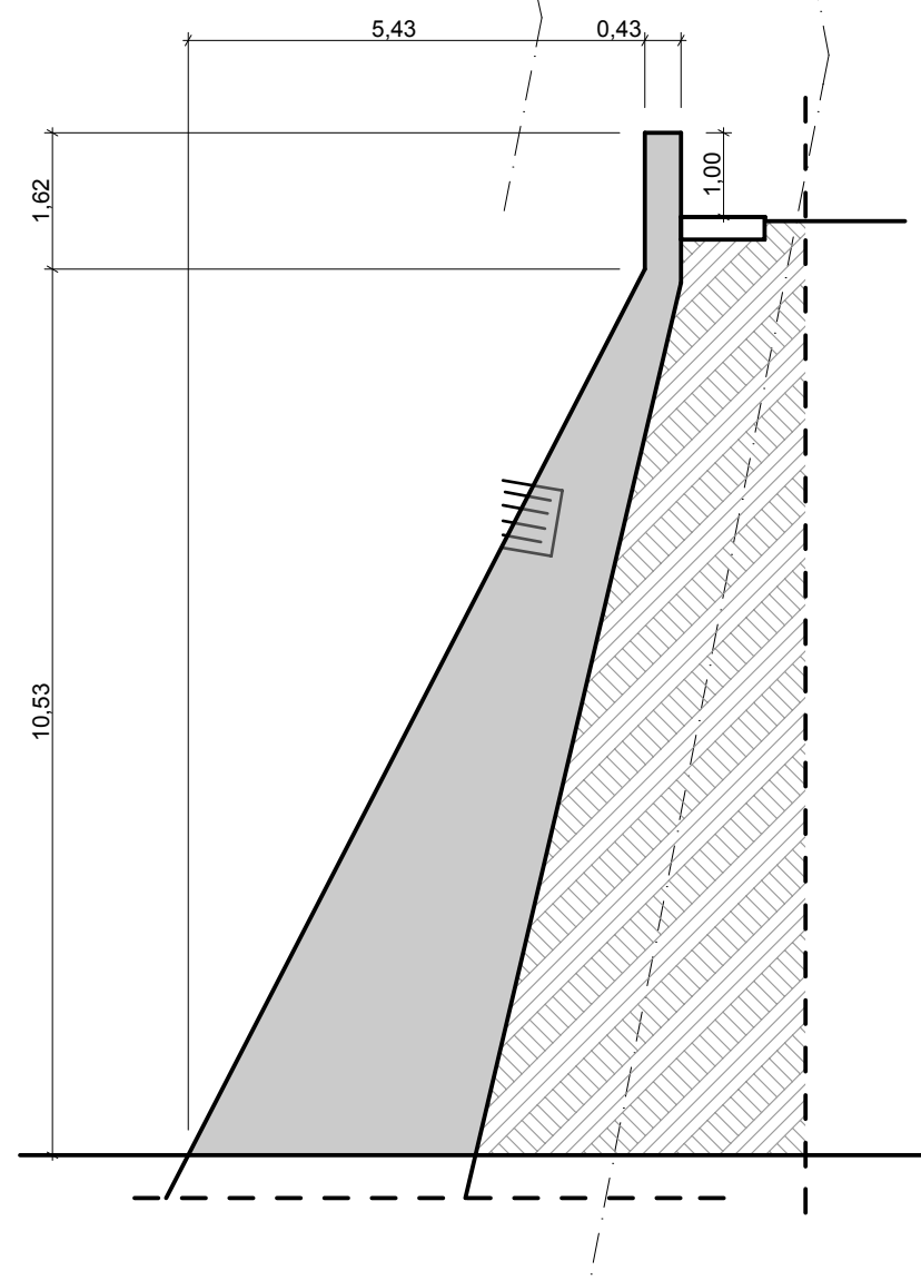
SEZIONE 8 - 8
