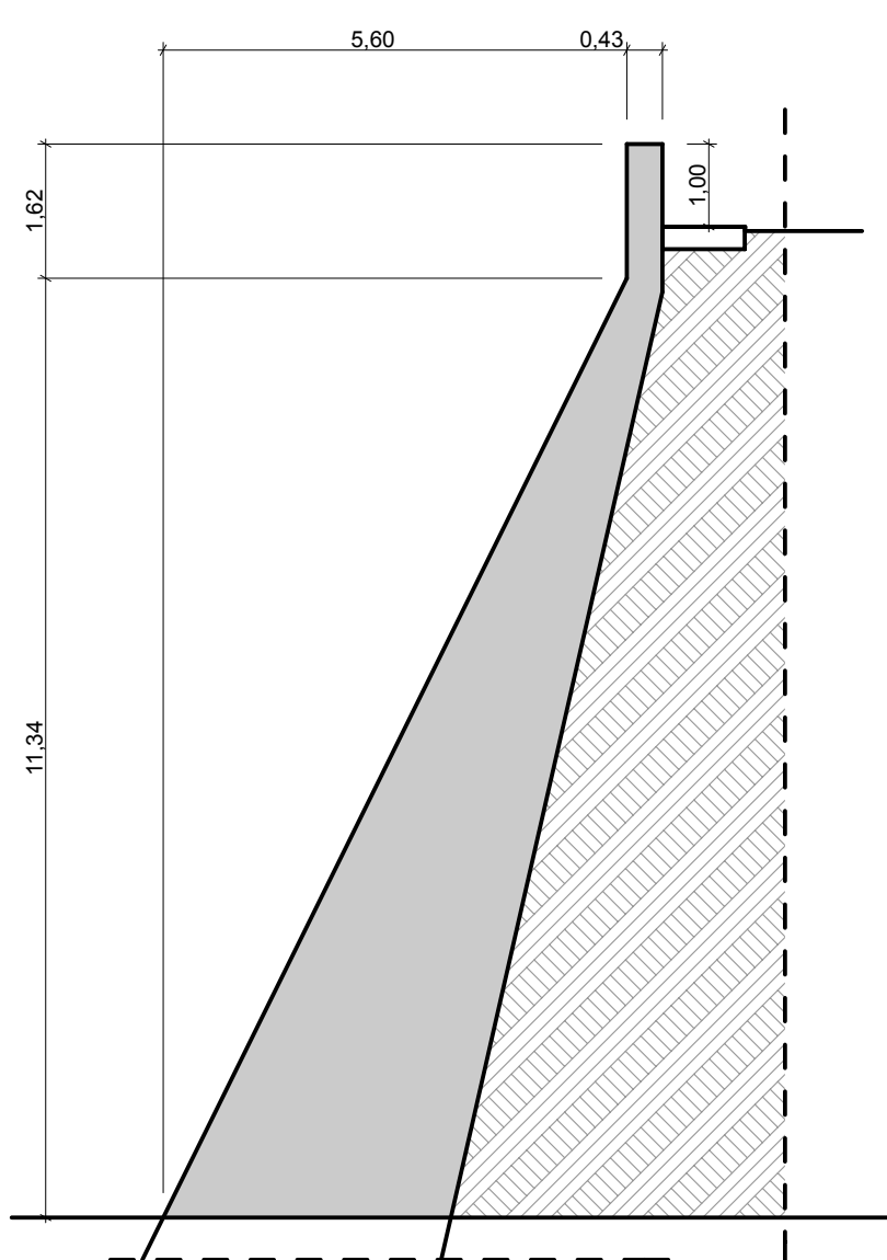
SEZIONE 5 - 5
