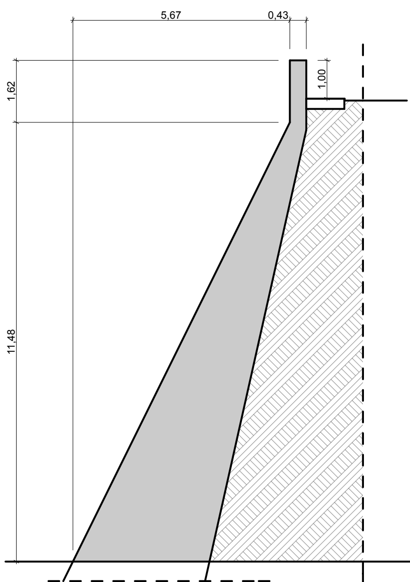
SEZIONE 6 - 6
