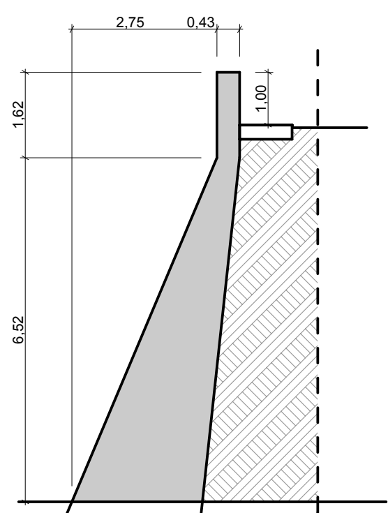
SEZIONE 2 - 2
