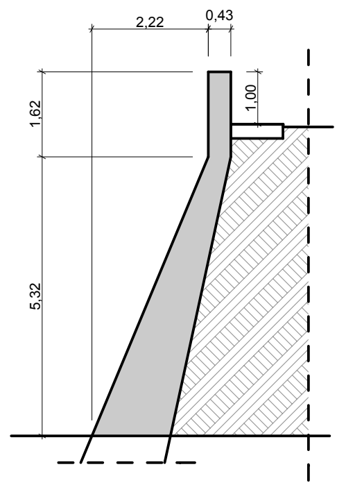
SEZIONE 1 - 1
