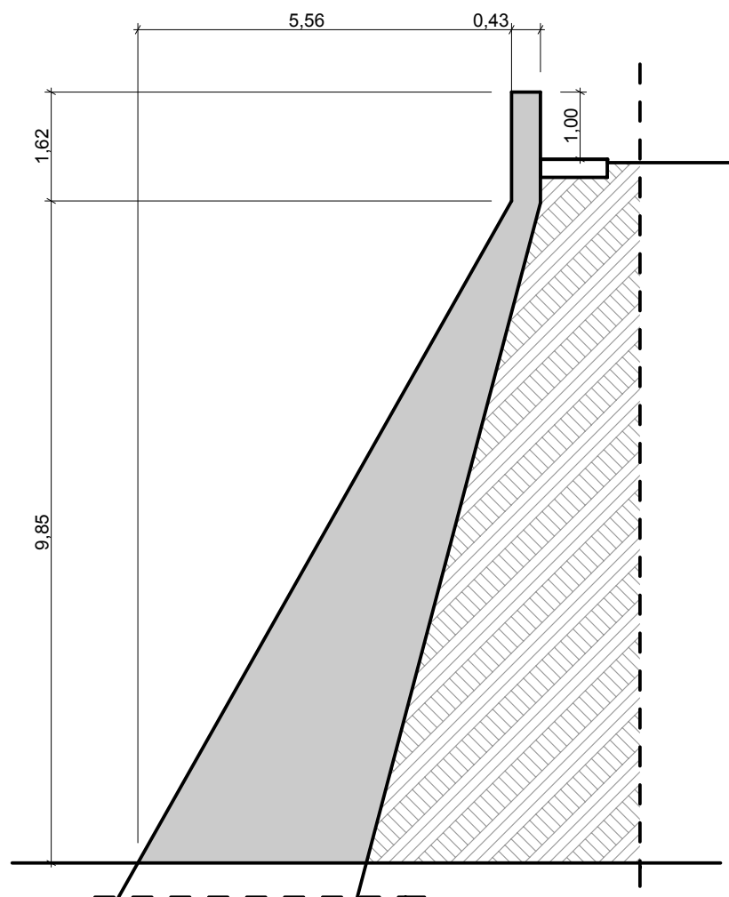
SEZIONE 3 - 3
