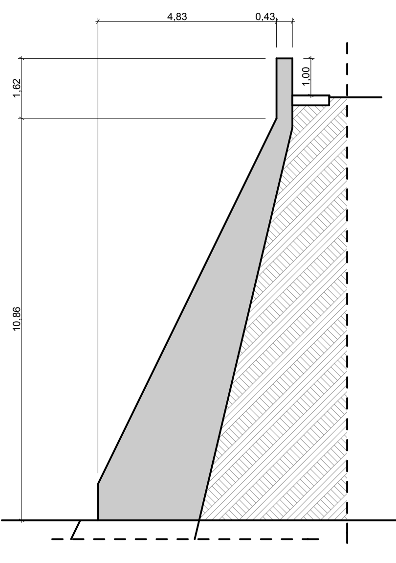
SEZIONE 7 - 7
