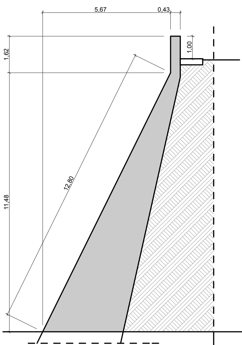
SEZIONE 6 - 6
