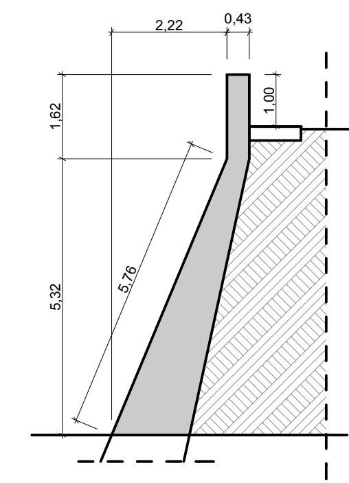
SEZIONE 1 - 1
