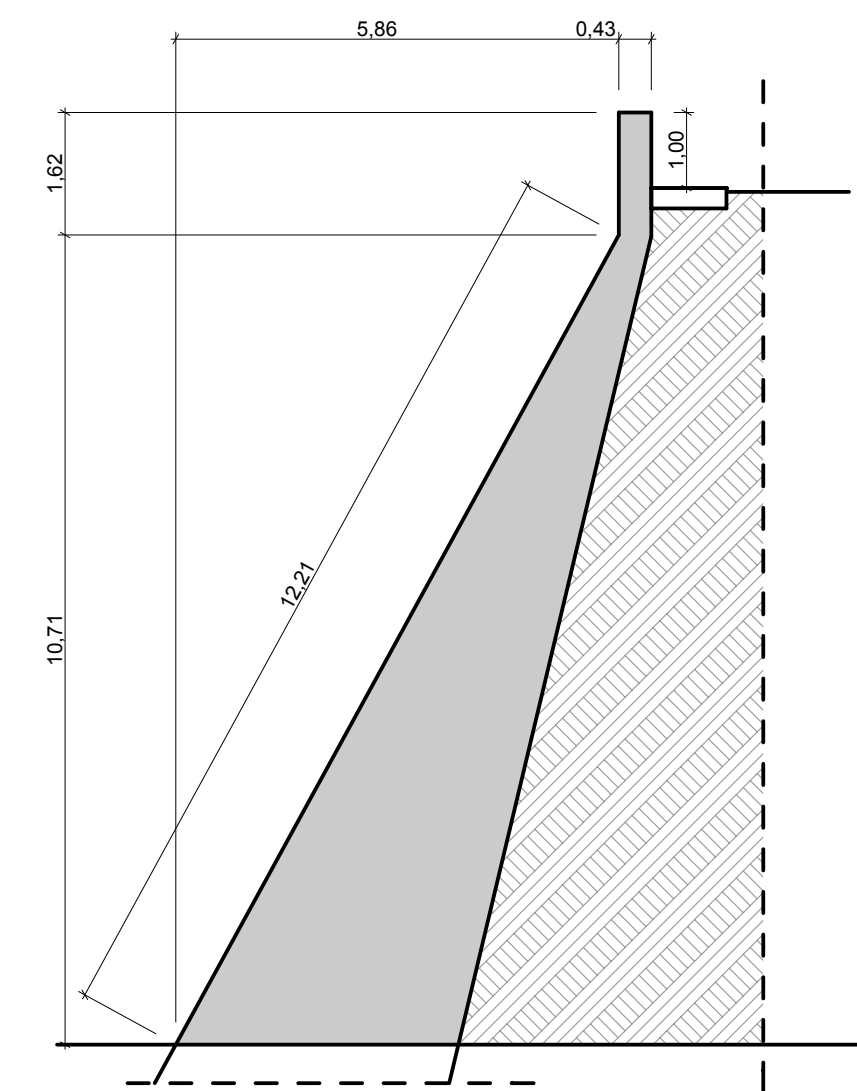
SEZIONE 4 - 4
