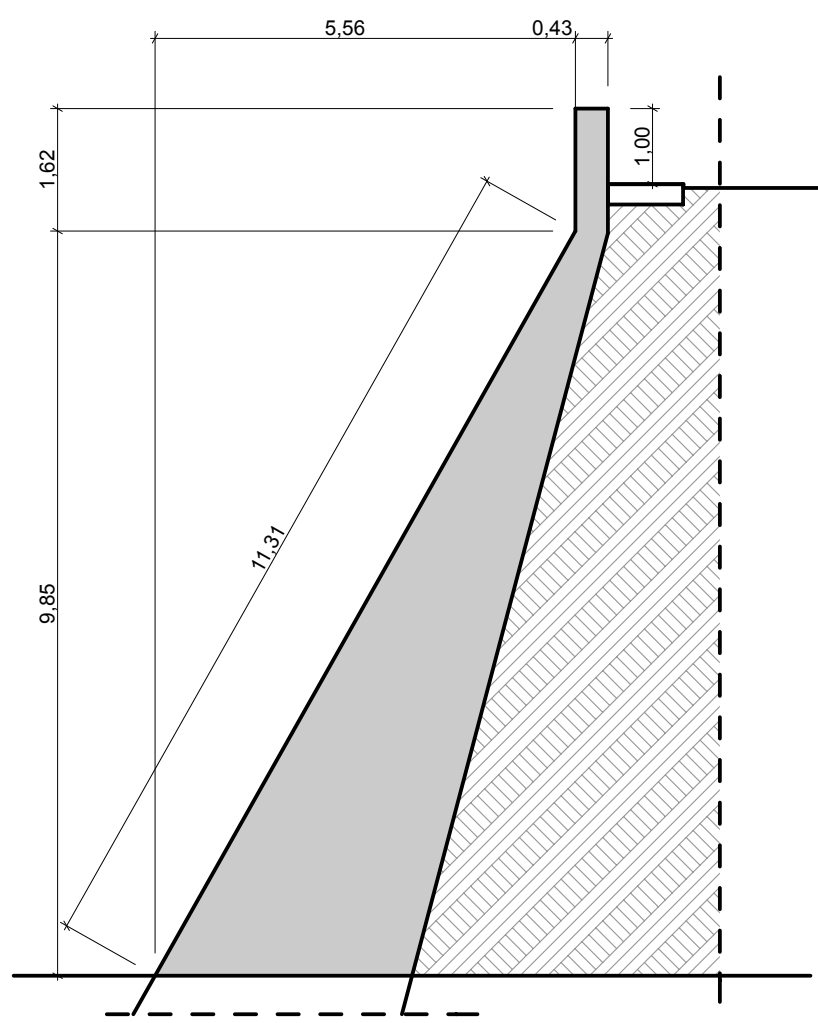
SEZIONE 3 - 3
