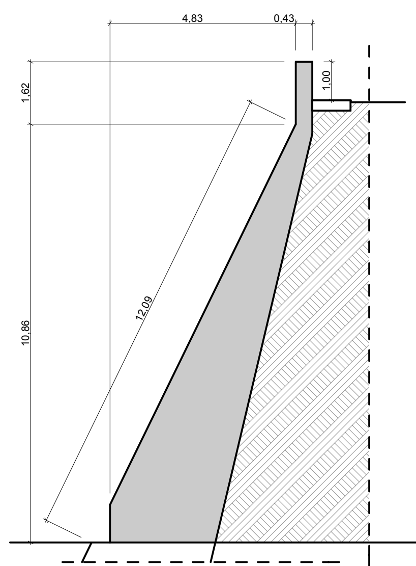
SEZIONE 7 - 7
