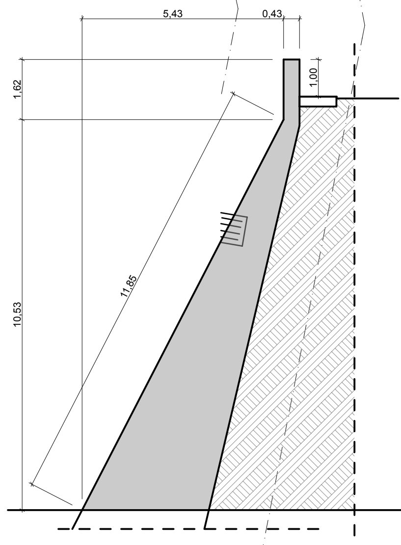
SEZIONE 8 - 8
