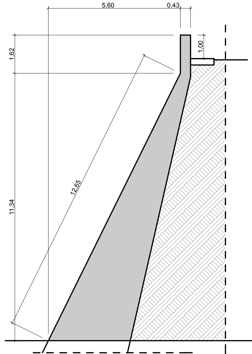
SEZIONE 5 - 5
