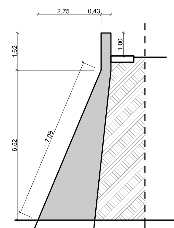
SEZIONE 2 - 2
