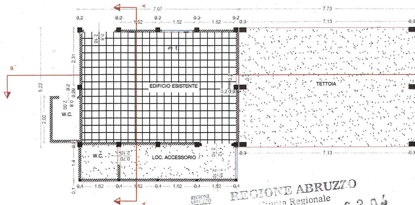
PIANTA 1:100
