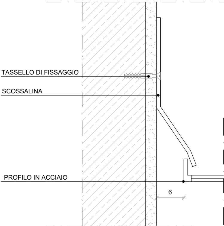
PARTICOLARE TIPO D: ANCORAGGIO PENSILINA-STRUTTURA ADIACENTE SCALA 1:5
