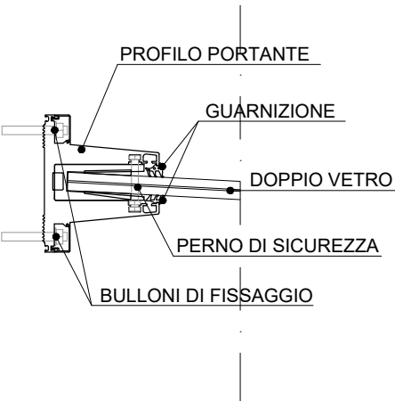
PARTICOLARE TIPO A: ANCORAGGIO PENSILINA- INFISSO SCALA 1:5
