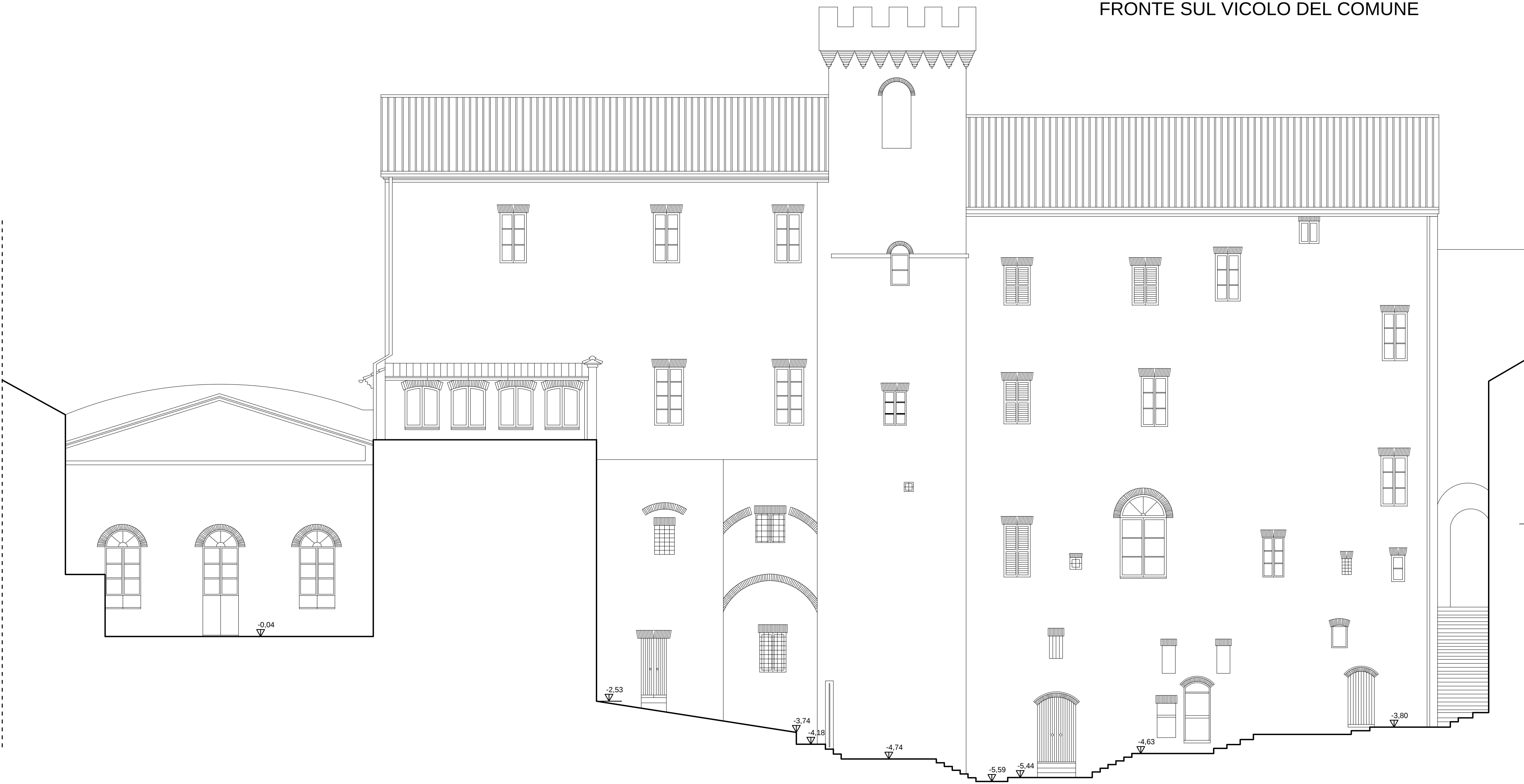
FRONTE SUL VICOLO DEL COMUNE
