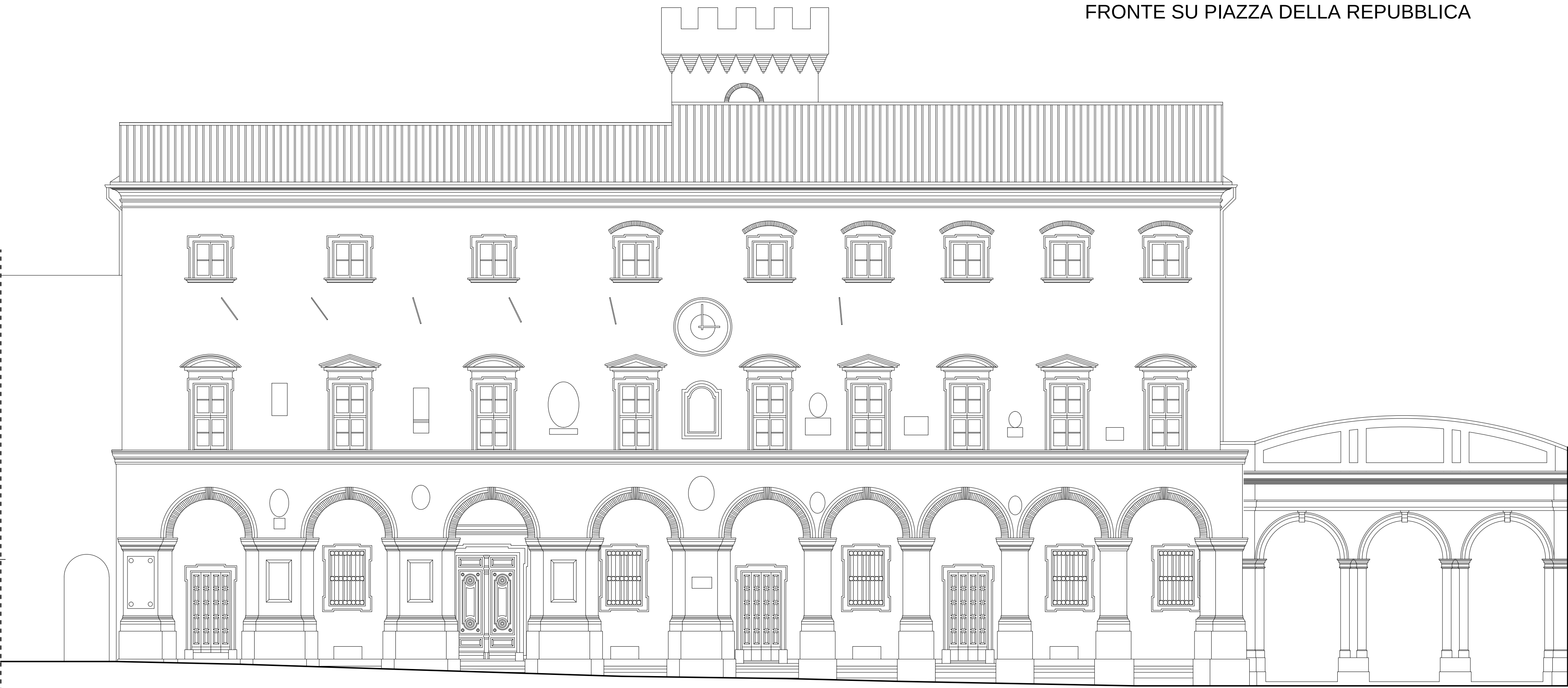
FRONTE SU PIAZZA DELLA REPUBBLICA
