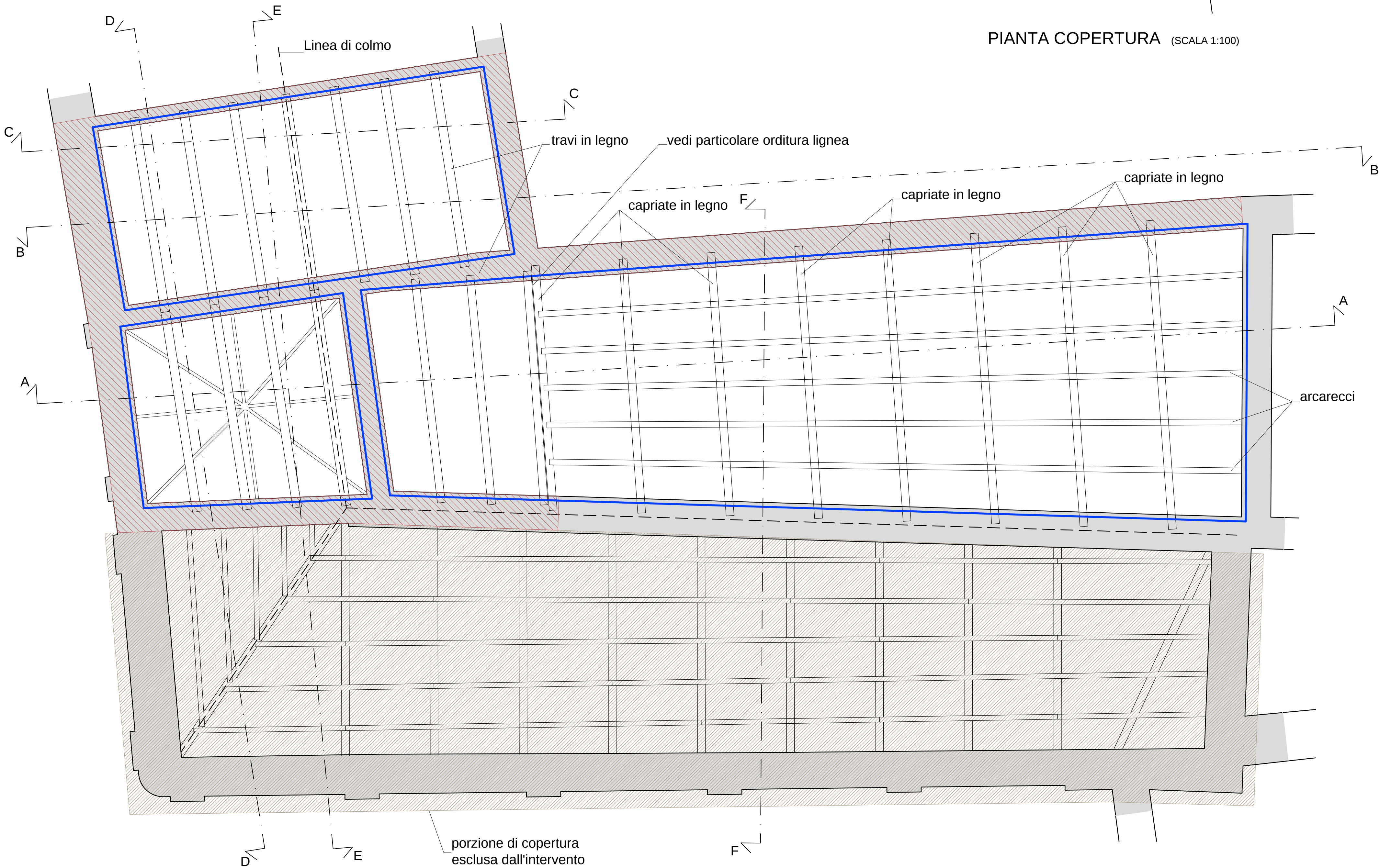
PIANTA ORDITURA LIGNEA
