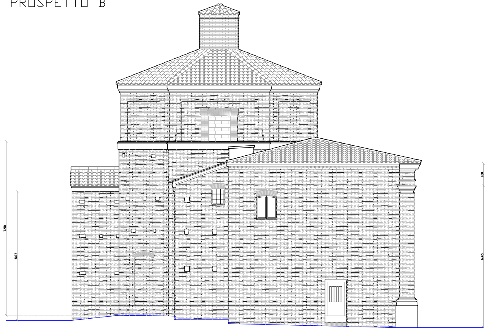
PROSPETTO B
