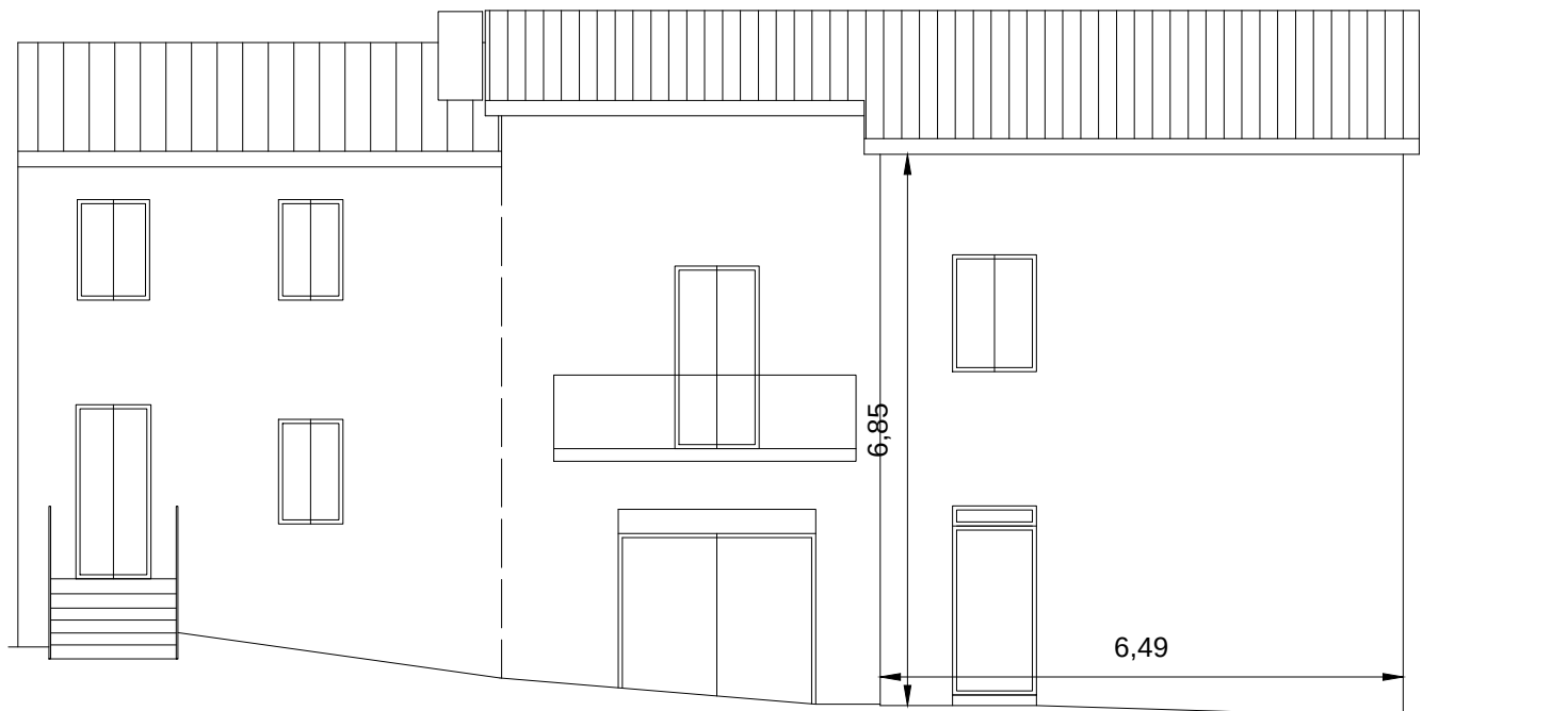
Prospetto Nord
