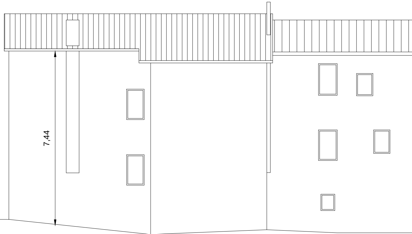
Prospetto Sud
