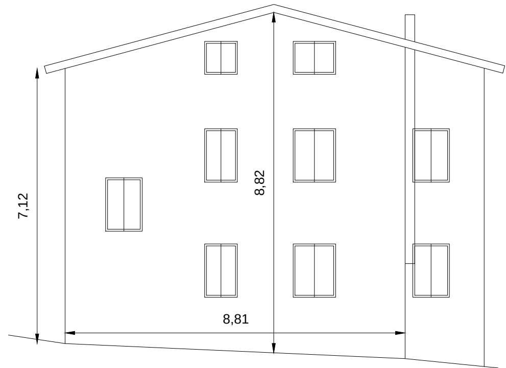
Prospetto Ovest
