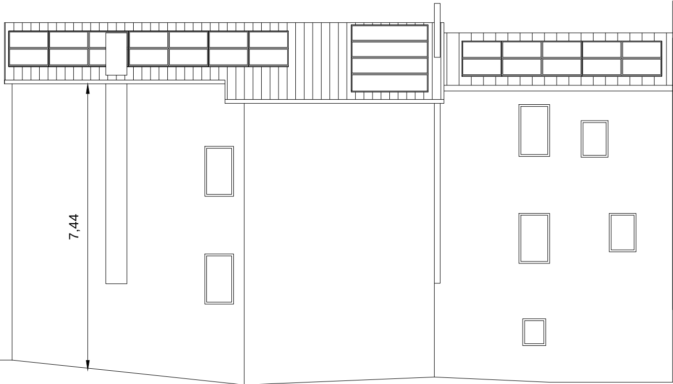
Prospetto Sud
