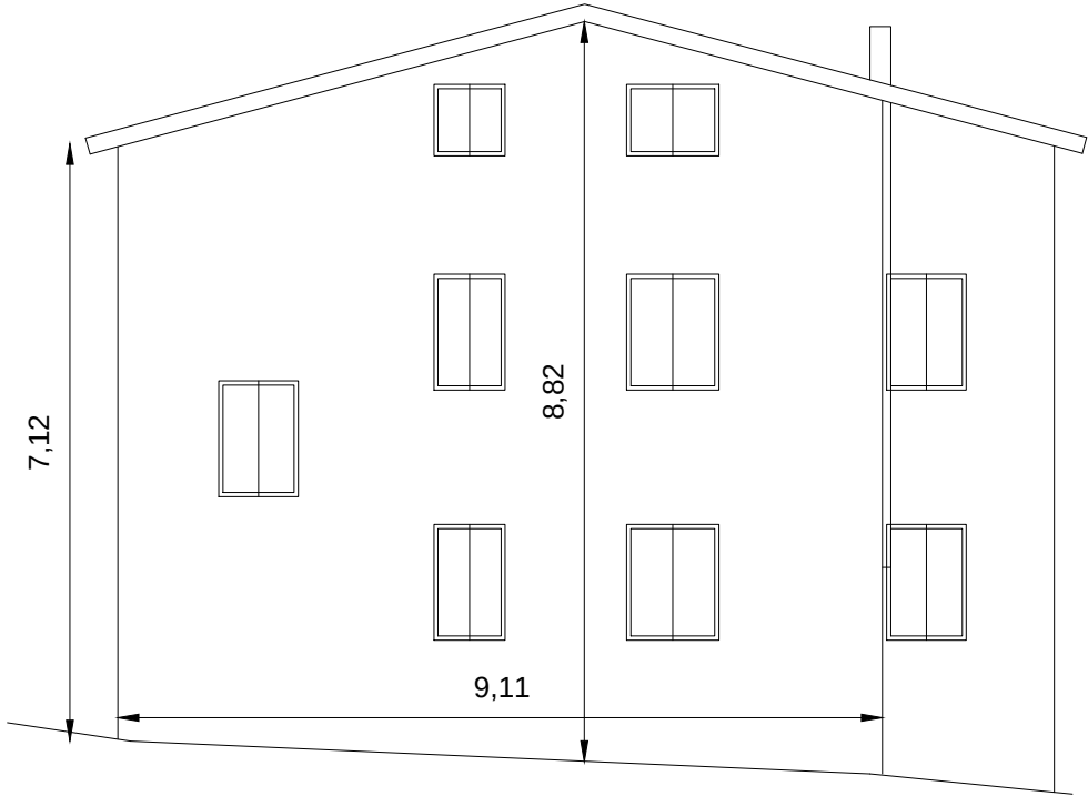
Prospetto Ovest
