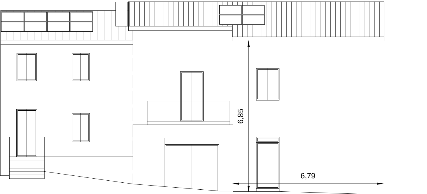
Prospetto Nord
