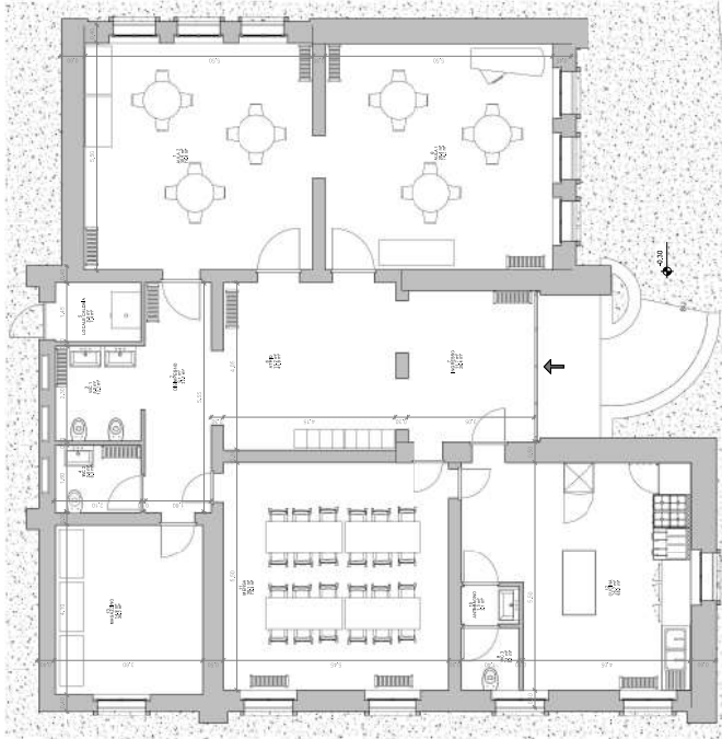
1 SP_ARCH_Pianta_PIANO_TERRA - Arredi e finiture 1:50
