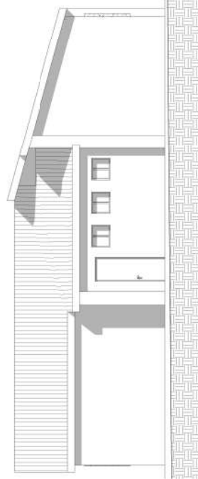
3 SP_ARCH_PROSPETTO_NORD - Stato finale 1:50
