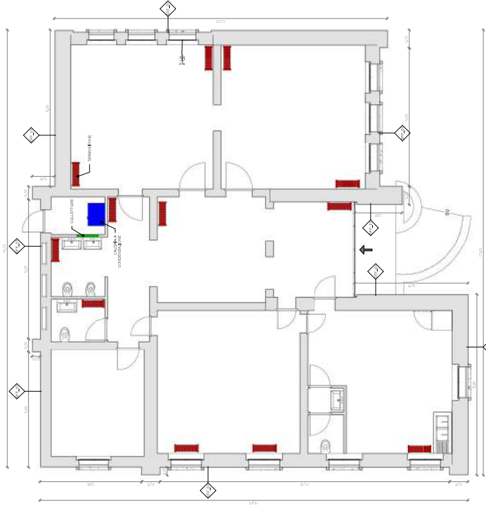
SP_EFF_PIANTA_IMPIANTO DI RISCALDAMENTO E APPARECCHI IDRAULICI
