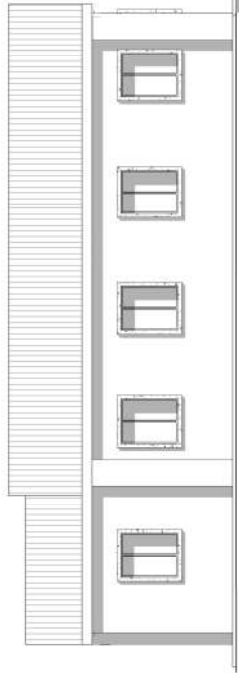
4 SP_ARCH_PROSPETTO_OVEST-Stato finale 1:50
