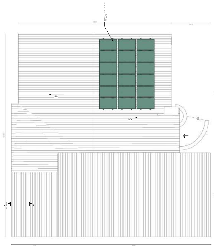
SP_EFF_DISPOSIZIONE IMPIANTO FOTOVOLTAICO
