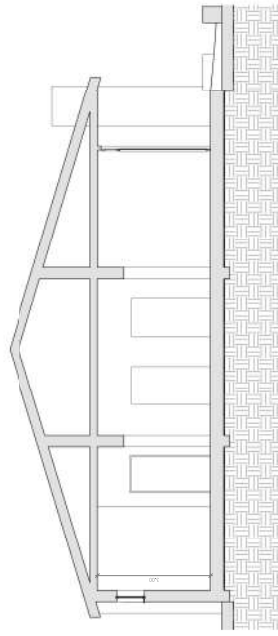
1-1 SF_ARCH_SEZIONE_1-1 1:50
