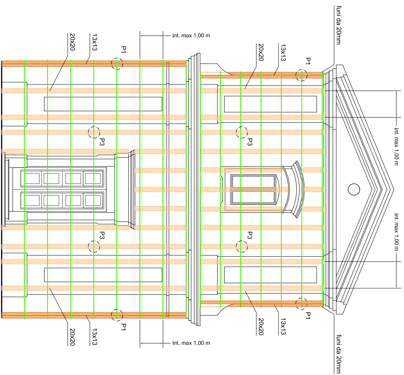
Prospetto principale
