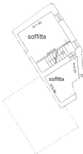
PIANTA PIANO SECONDO
