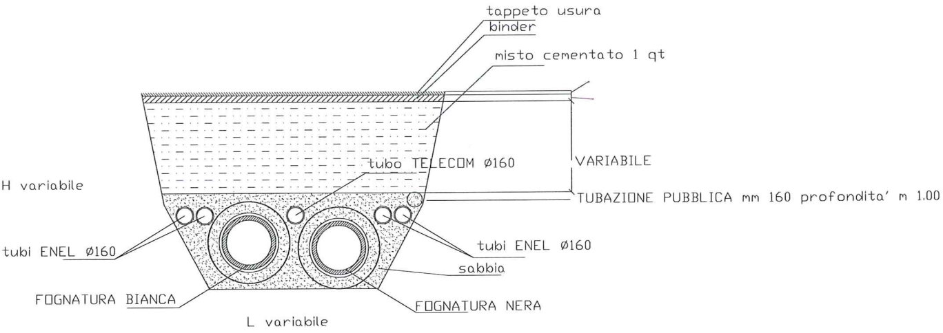
SEZIONE DI SCAVO TIPO SU STRADA ASFALTATA tratto N5-N7 SAE
