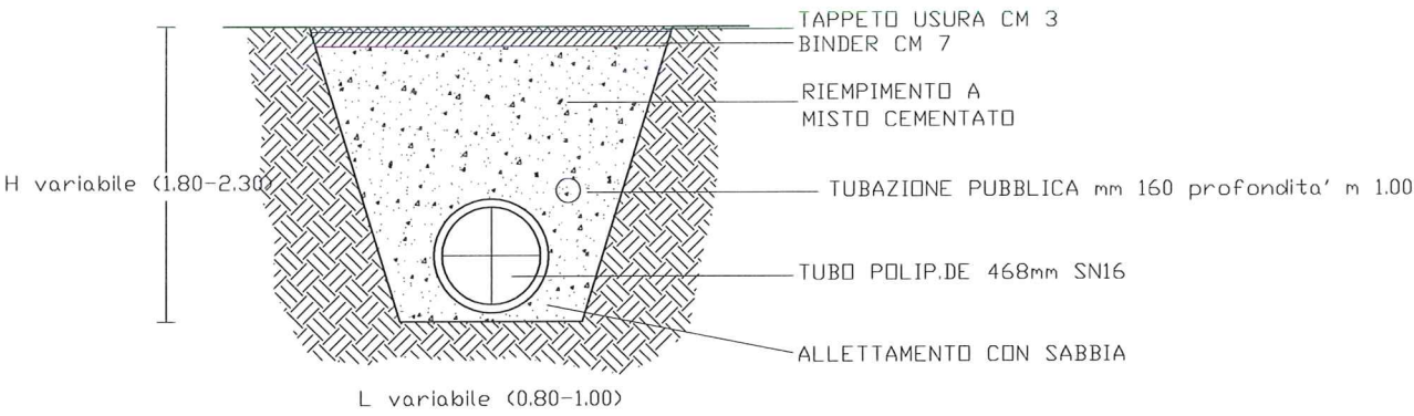
SEZIONE DI SCAVO TIPO SU STRADA ASFALTATA tratto N1-N5
