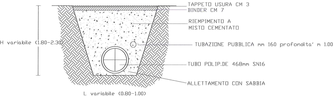
SEZIONE DI SCAVO TIPO SU STRADA ASFALTATA tratto N7-N10
