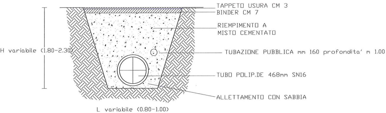
SEZIONE DI SCAVO TIPO SU STRADA ASFALTATA tratto attraversamento
