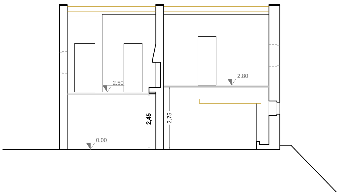
Sezione B-B'
