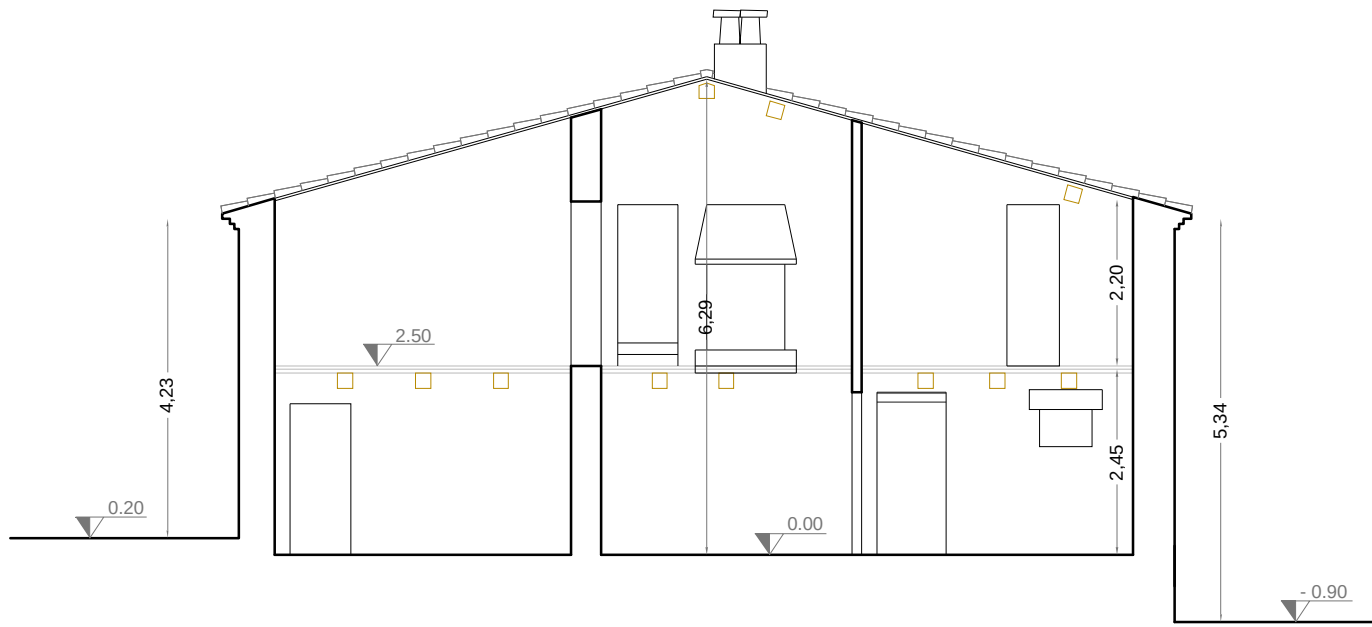
Sezione A-A'
