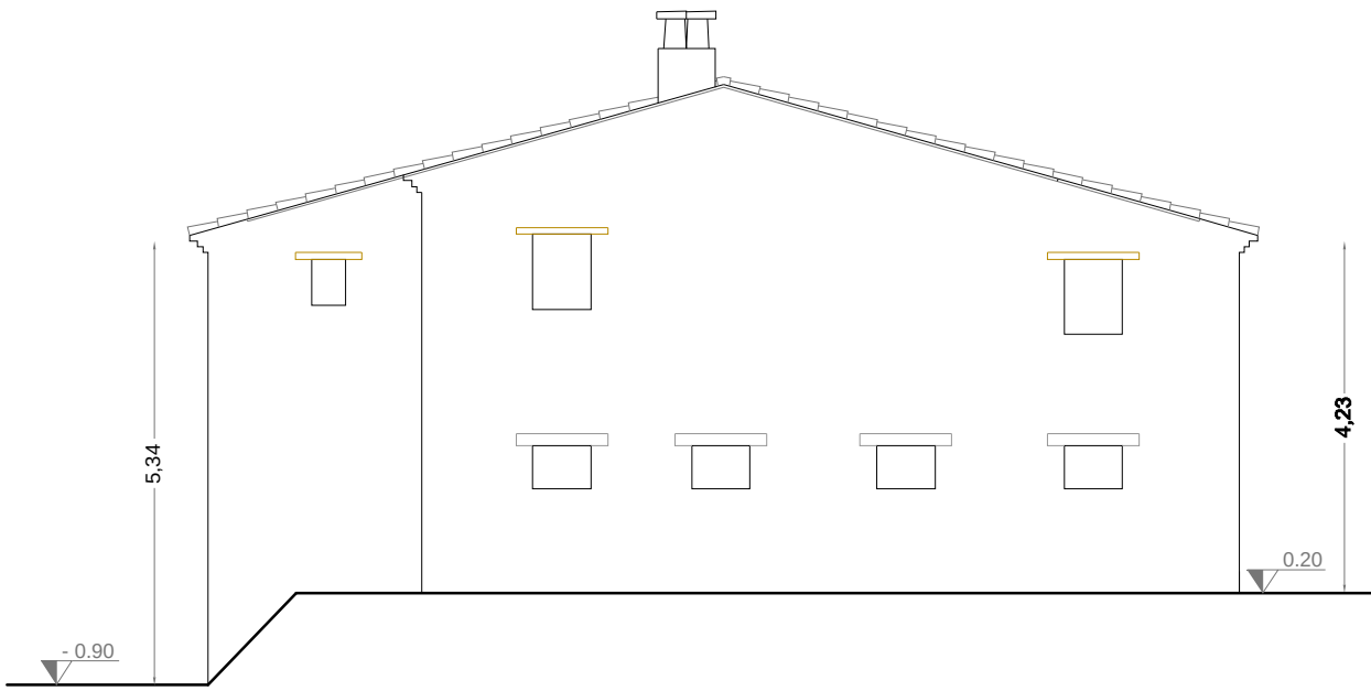
Prospetto ovest
