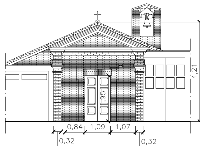
PROSPETTO EST SC 1/100
