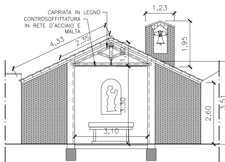
SEZIONE A-A' SC 1/100
