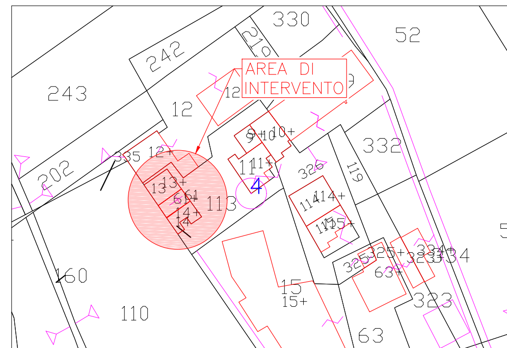
STRALCIO CATASTALE SC 1/1000
