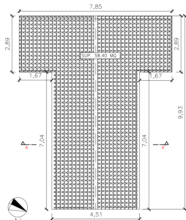
PIANTA COPERTURA SC 1/100
