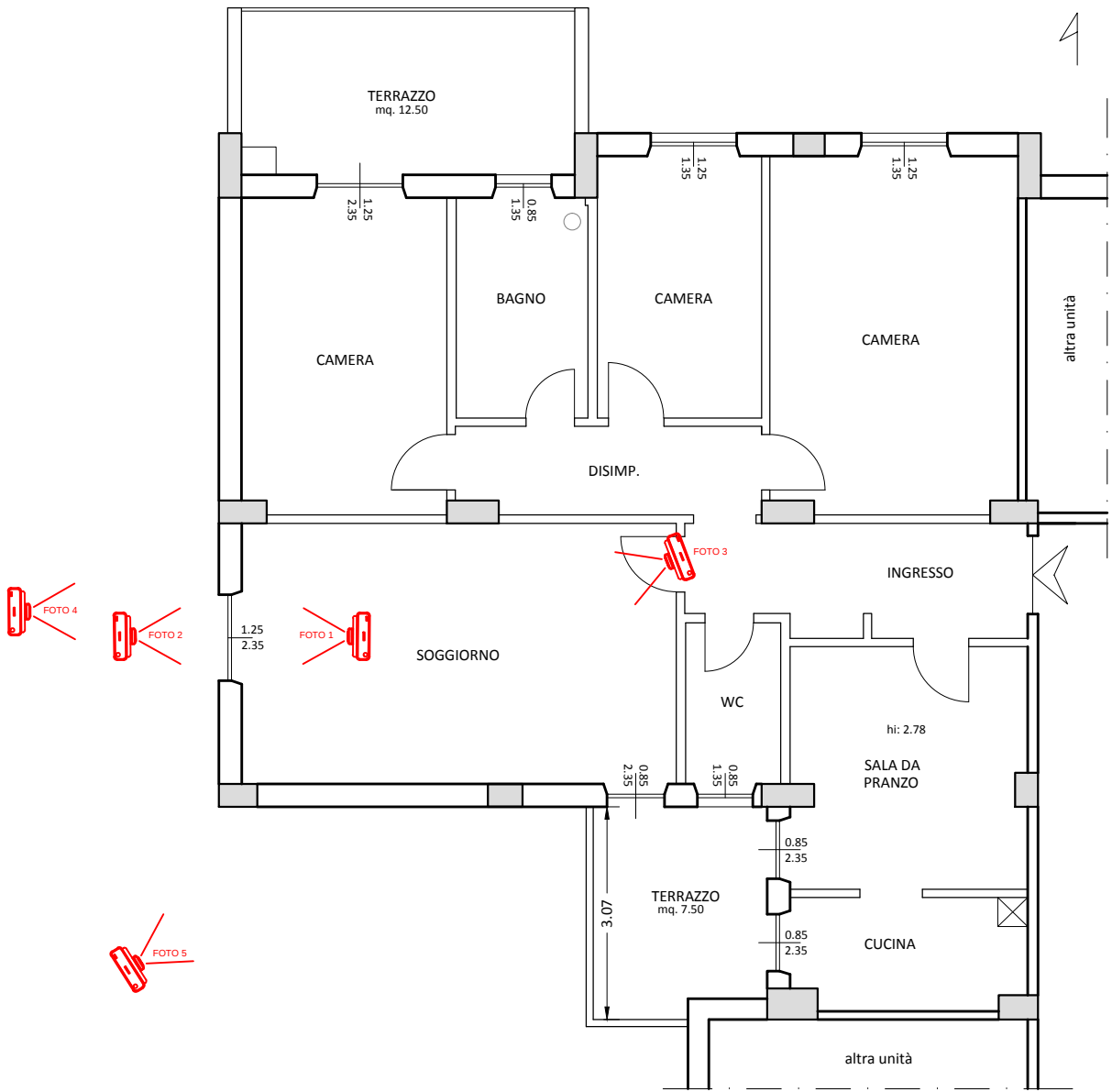
PIANTA STATO ATTUALE SC. 1:100
