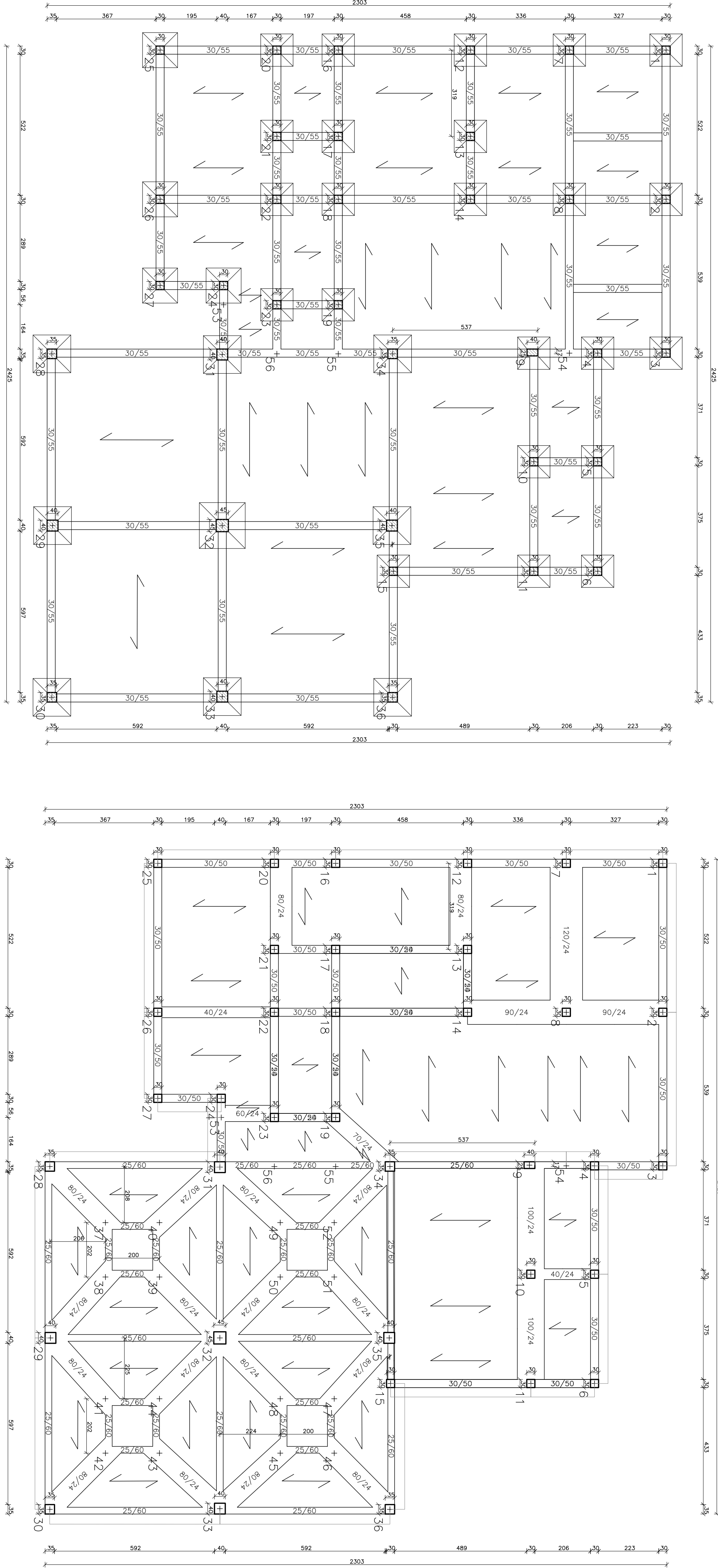
pianta IMPALCATO QUOTA 0.00m
