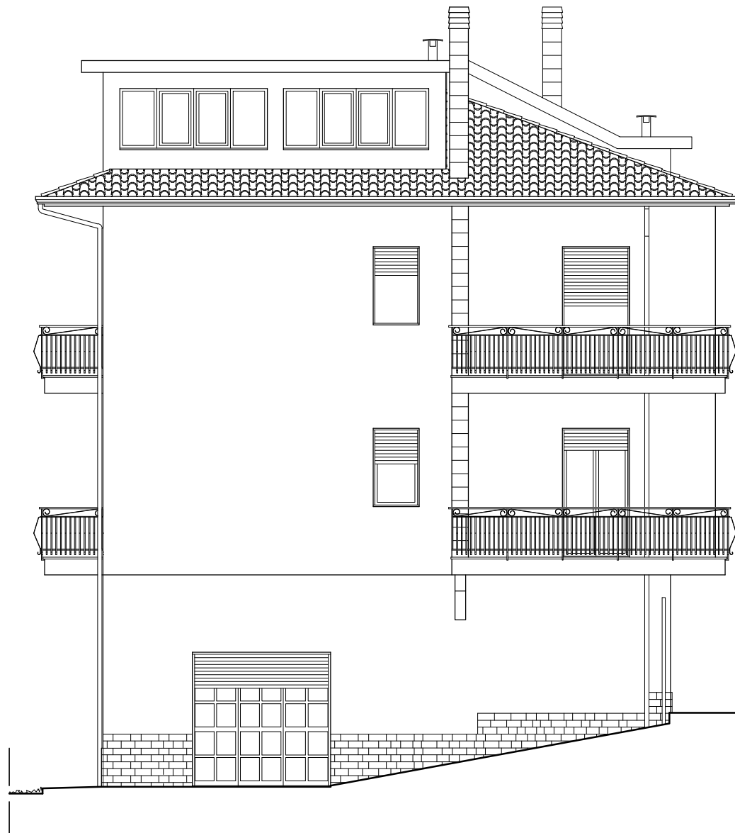
PROSPETTO EST
