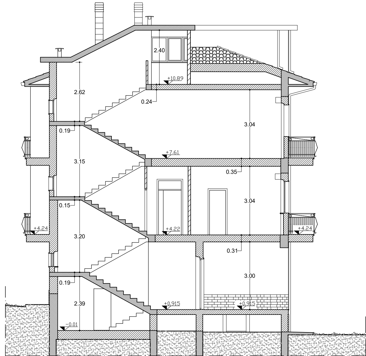
SEZIONE A - A
