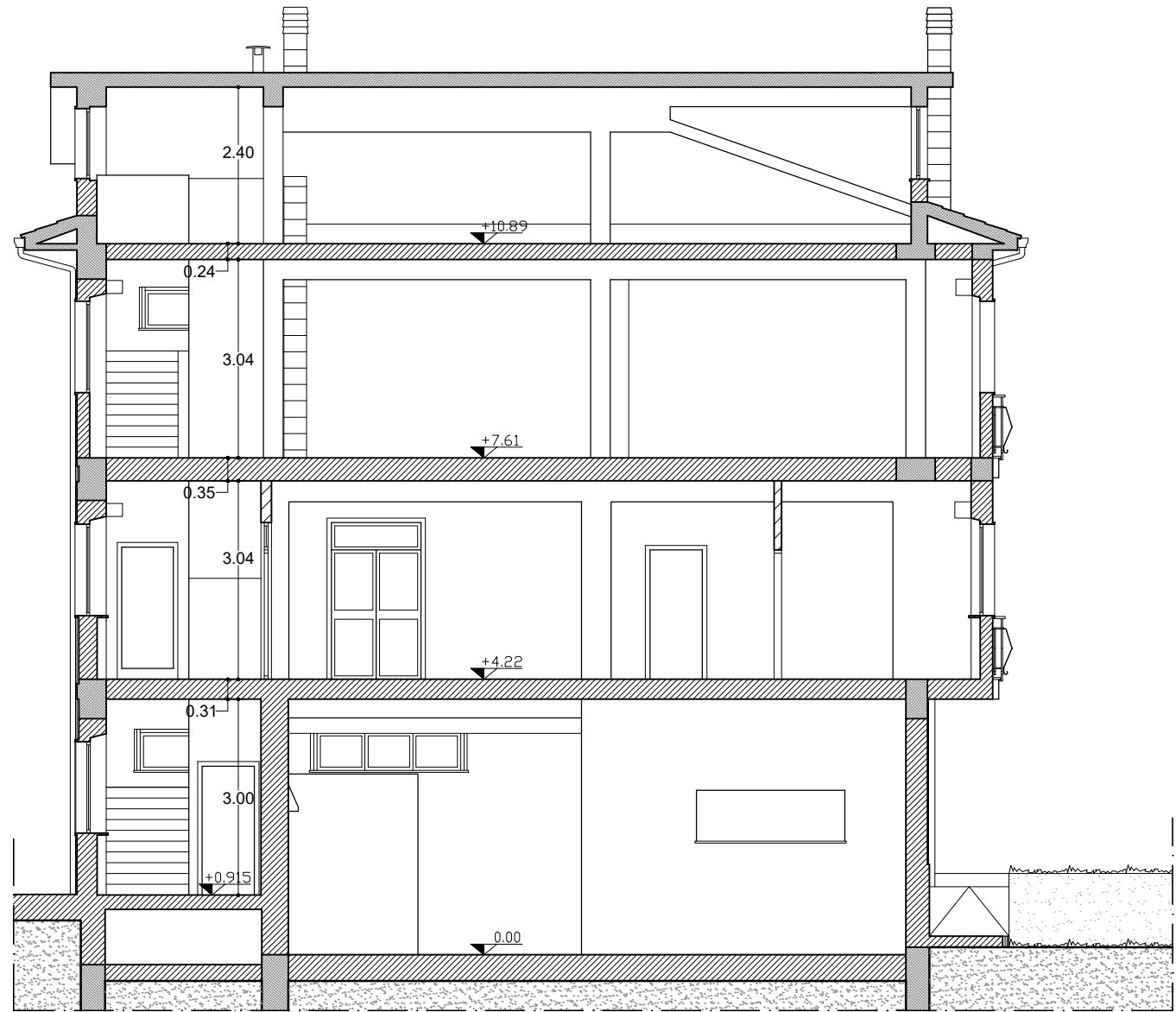
SEZIONE B - B
