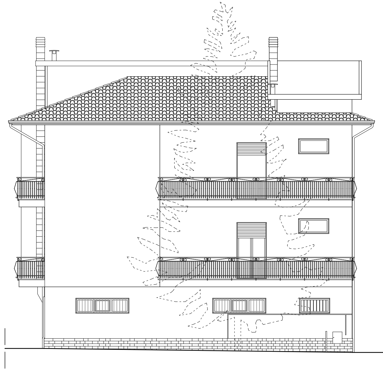
PROSPETTO EST
