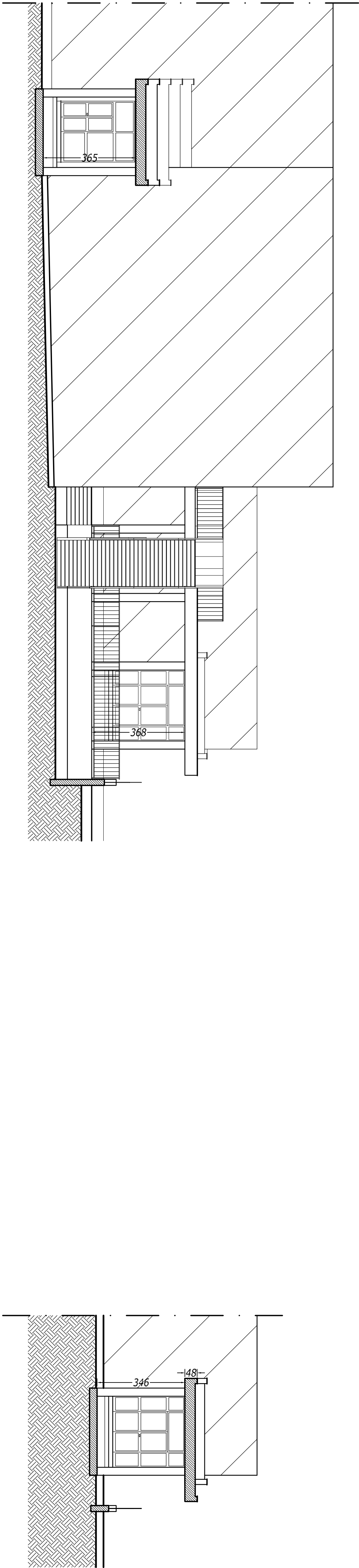
SEZIONE A-A
