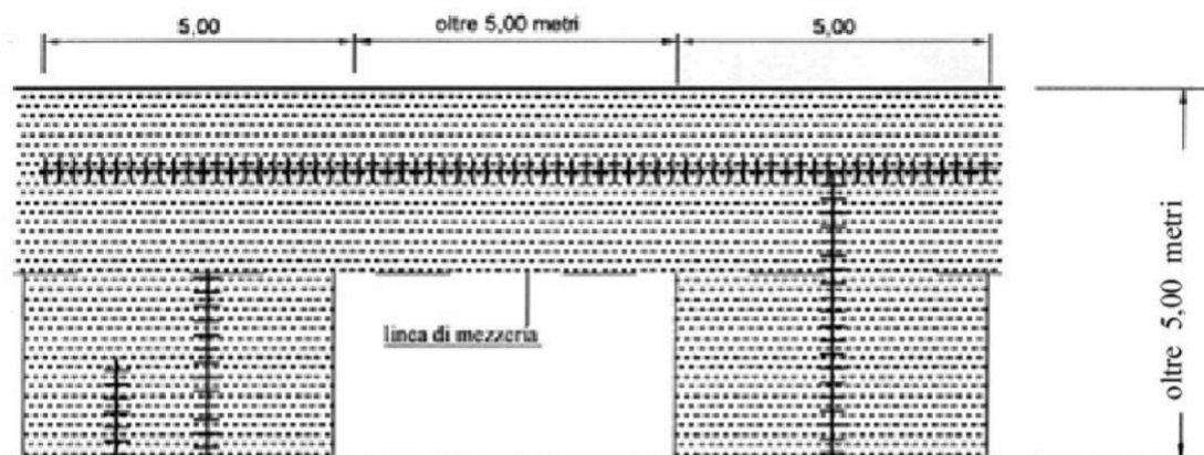
figura 13 scavi multipli
