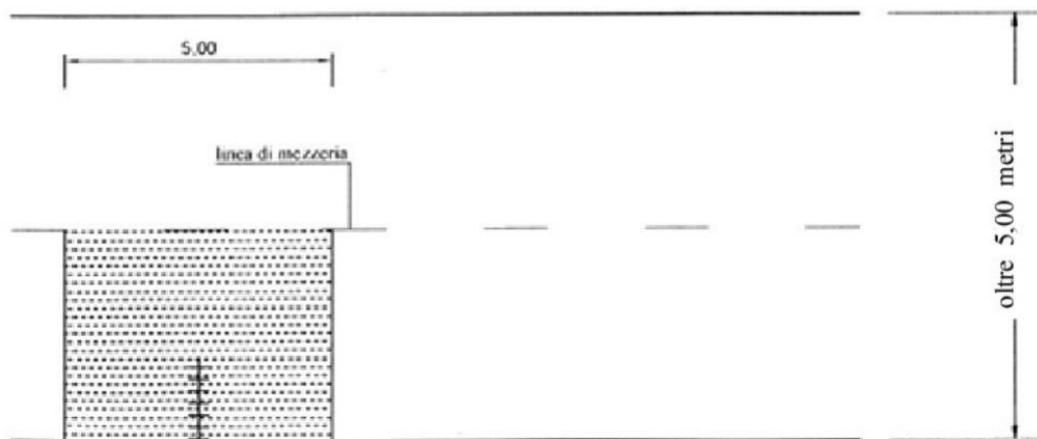
figura 8 scavo trasversale alla carreggiata
