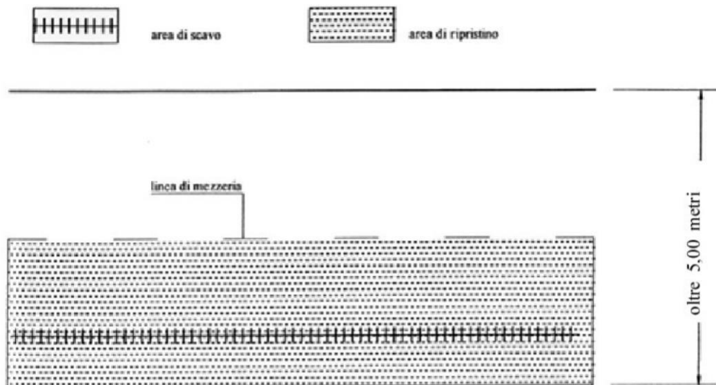
figura 7 scavo longitudinale alla carreggiata
