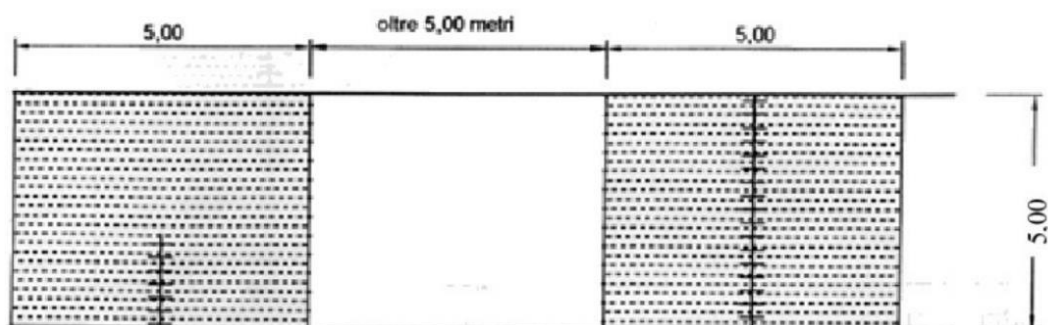
figura 6 scavi multipli
