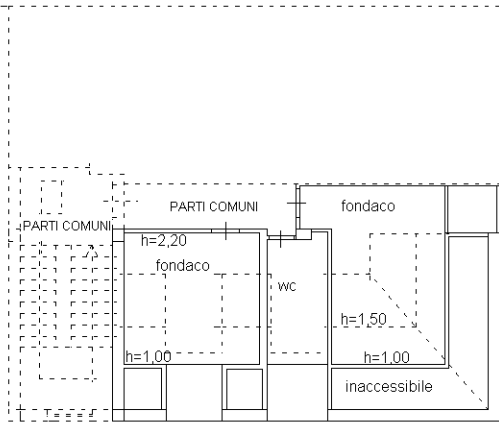
Piano terzo (sottotetto)
