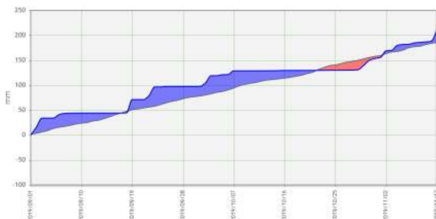
Fig. 1. Linea blu: precipitazione giornaliera cumulata 1 settembre – 12 novembre 2019 (mm). Linea grigia: precipitazione giornaliera cumulata di riferimento 1981-2010 (mm). Le bande blu indicano periodi più piovosi con cumuli di precipitazione superiori alla media 1981-2010. Allo stesso modo, le bande rosse indicano periodi più secchi con precipitazioni al di sotto della norma.
