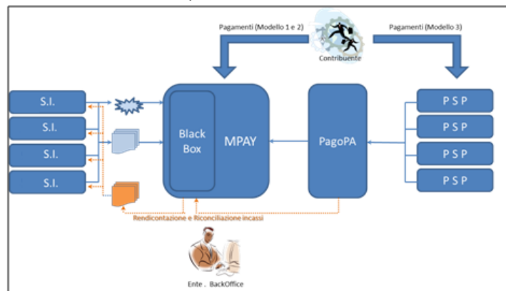
Figura 7 - Interoperabilità dei sistemi
