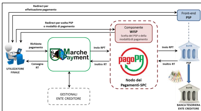
Figura 9 - Modalità di integrazione
