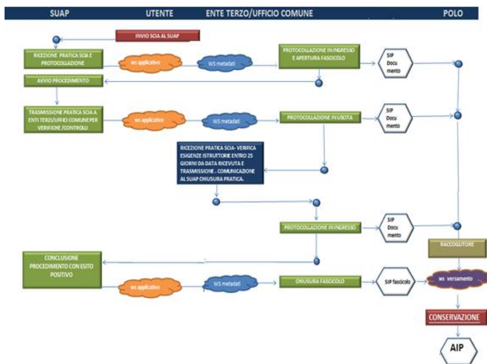
Figura 13 - Architettura integrazione SUAP/SUE
