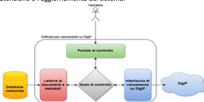
Figura 12 - Architettura funzionale integrazione Halley
