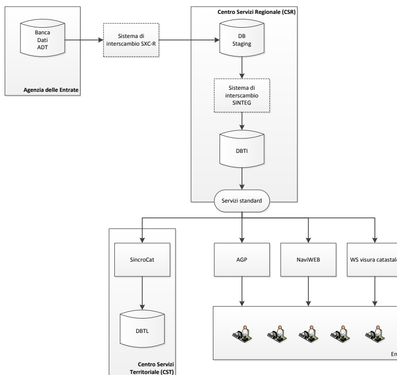
Figura 14 - Architettura funzionale SigmaTER
