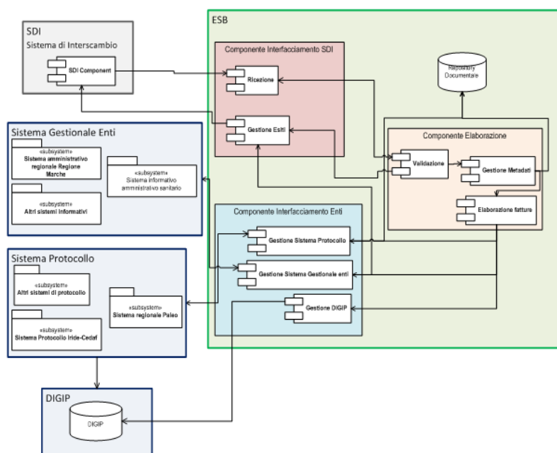
Figura 11 – Architettura tecnica di riferimento – da Regione Marche
