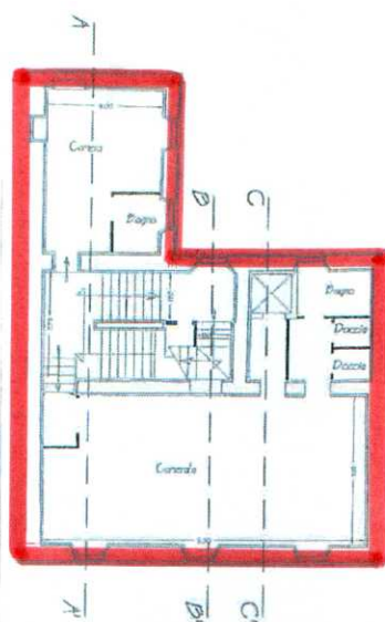
Pianta piano secondo
