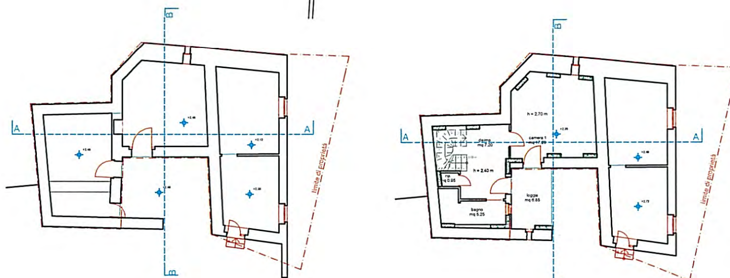
PIANO PRIMO ATTUALE
