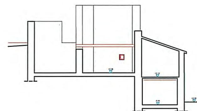
SEZIONE A-A ATTUALE
