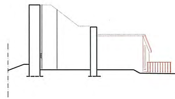
SEZIONE B-B ATTUALE
