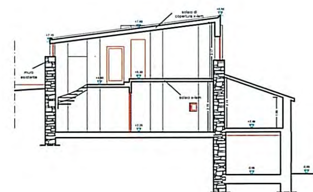
SEZIONE A-A MODIFICATA
