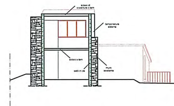
SEZIONE B-B MODIFICATA
