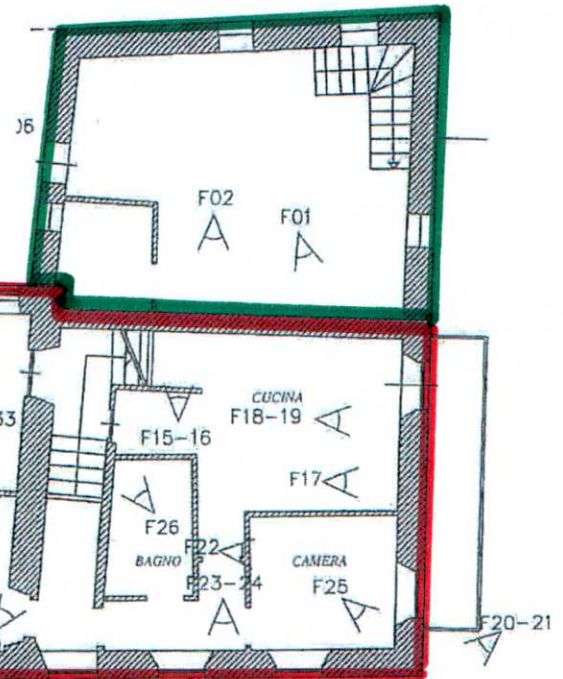
PIANO PRIMO
