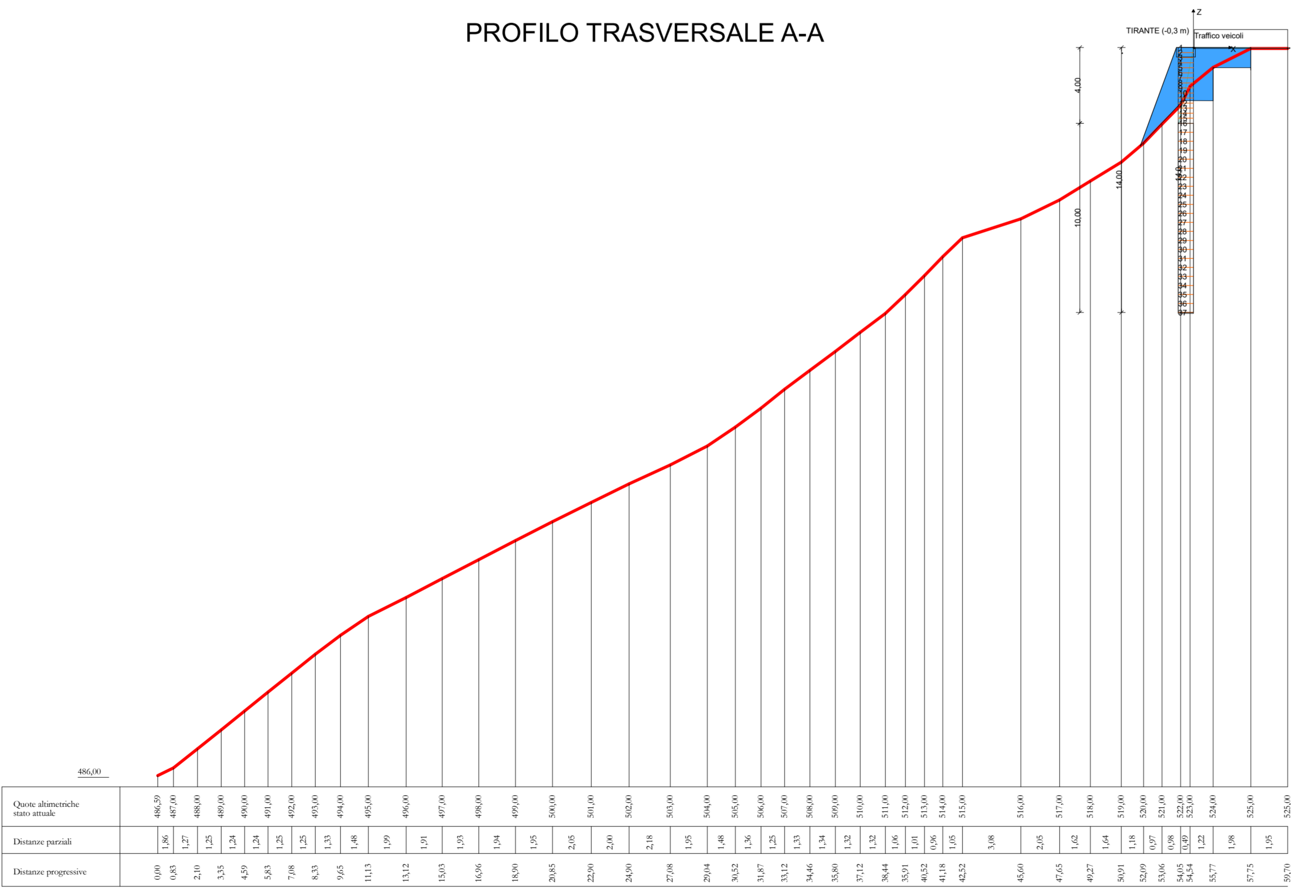
PROFILO TRASVERSALE A-A
