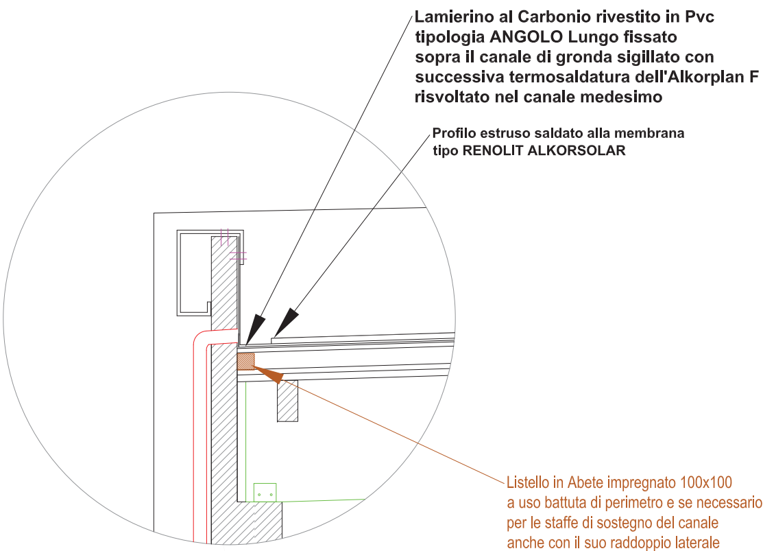
Profilo estruso saldato alla membrana tipo RENOLIT ALKAORSOLAR
