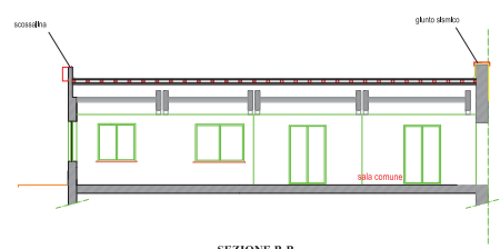
SEZIONE B-B
