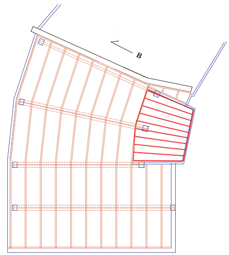
Correnti in legno 10x10
