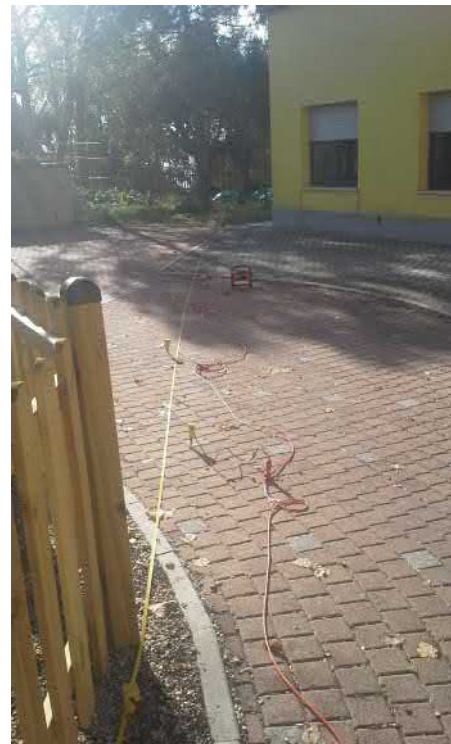
Stesa sismica attiva MASW
