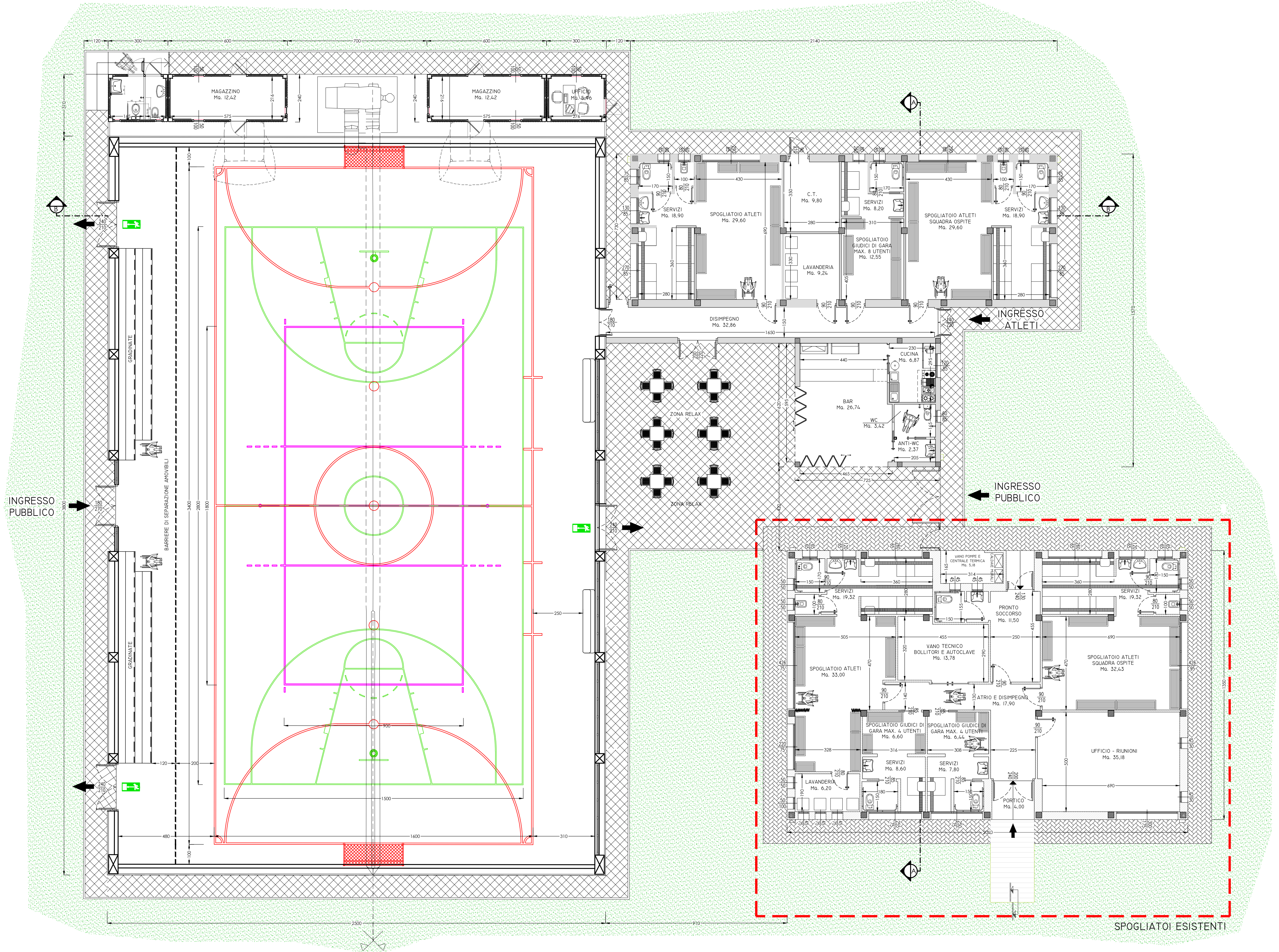
PIANTA PIANO TERRA (1:200)
