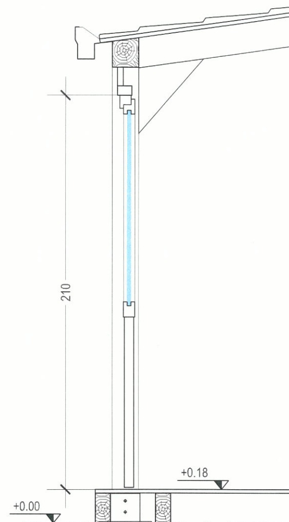
SEZIONE "C" Porta di ingresso
