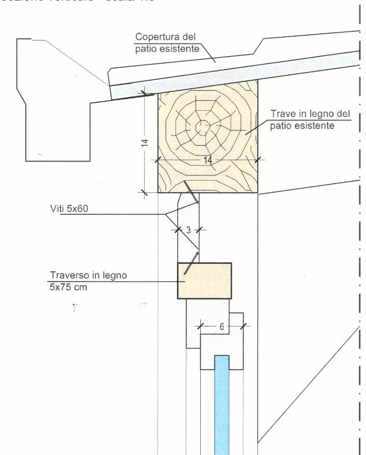
ATTACCO SUPERIORE SISTEMA BLOCK BAU sezione verticale - scala 1:5
