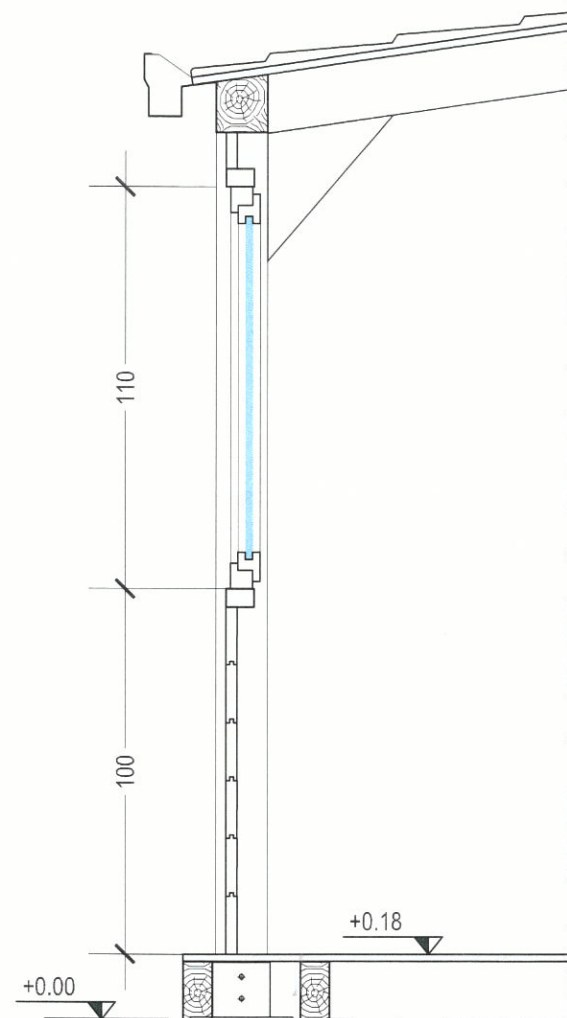
SEZIONE "B" Finestra apribile
