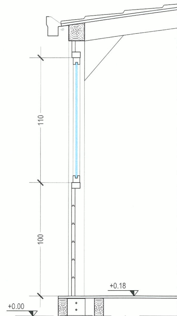
SEZIONE "A" Vetratura fissa
