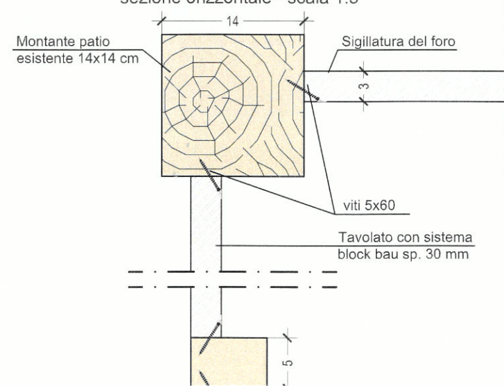
ATTACCO LATERALE SISTEMA BLOCK BAU sezione orizzontale - scala 1:5
