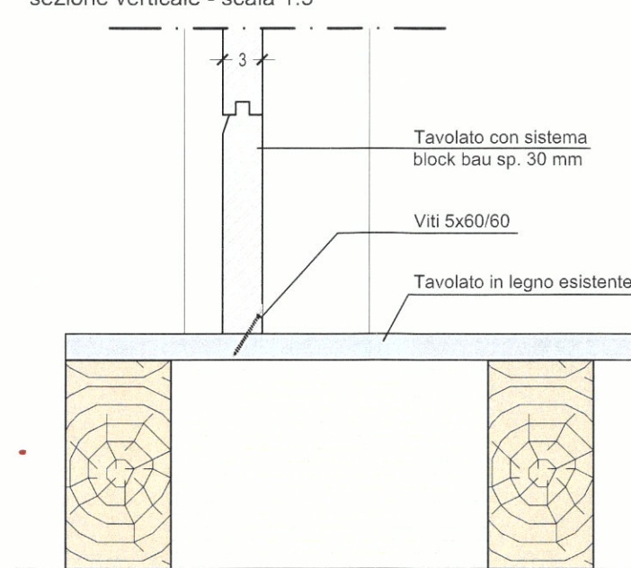
ATTACCO A TERRA SISTEMA BLOCK BAU sezione verticale - scala 1:5
