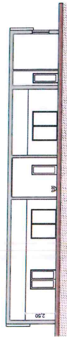
SEZIONE LONGITUDINALE
